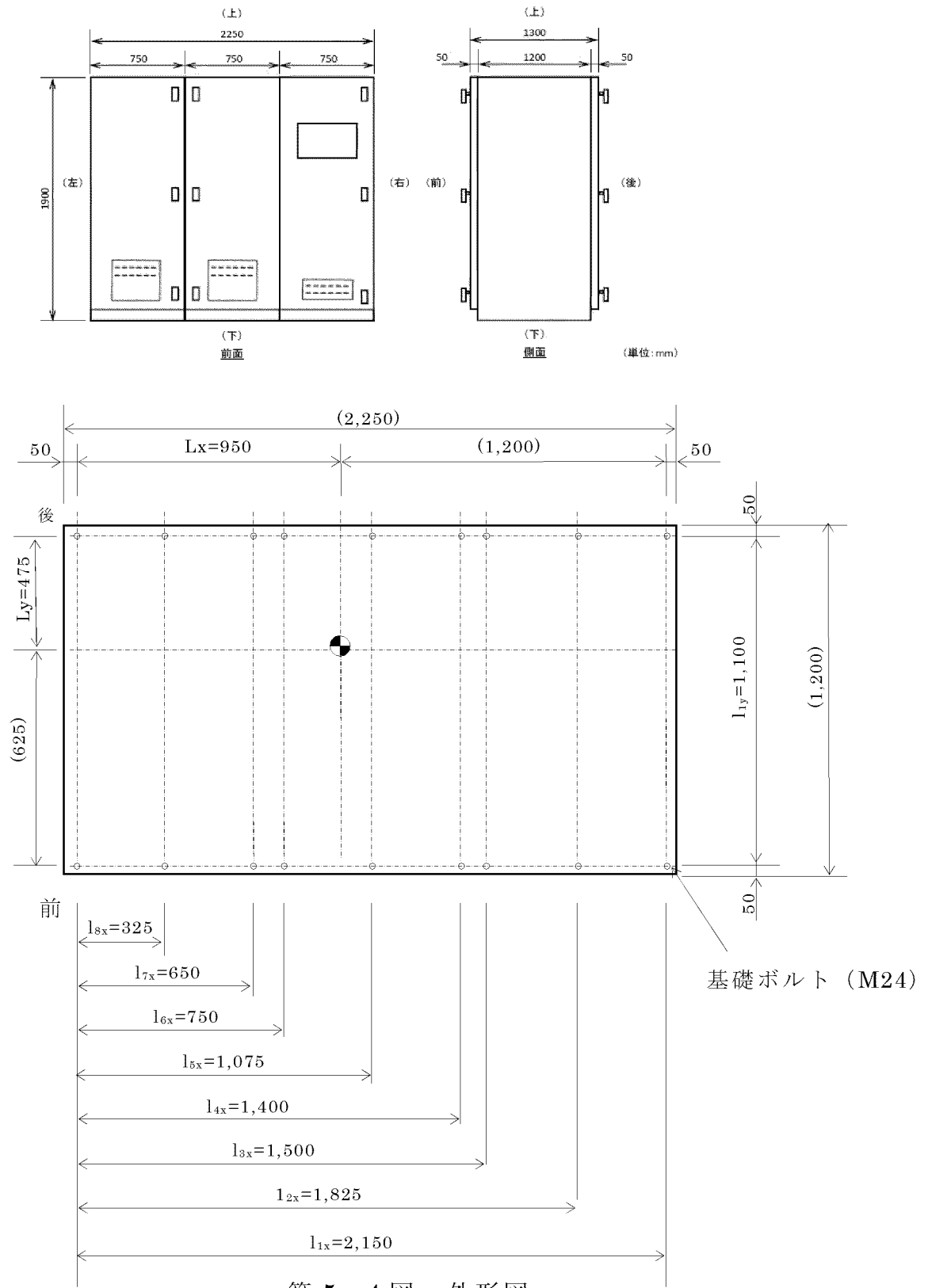
第 5-4 図 外形図
