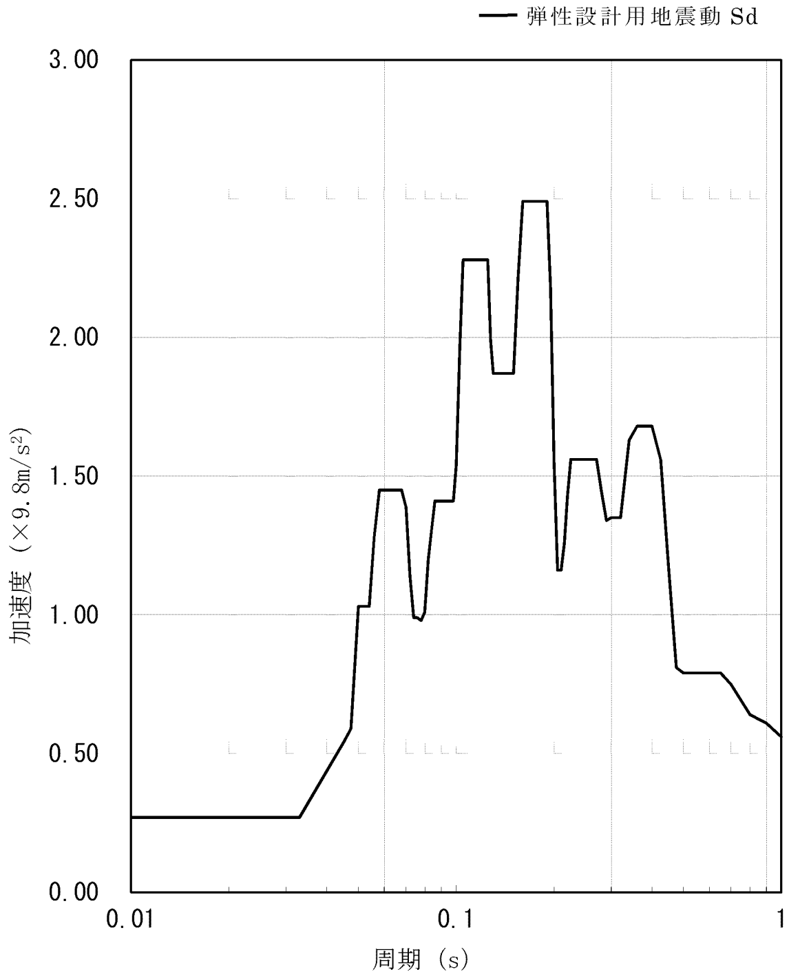
第 5-2 図(2/2) 弾性設計用地震動 Sd (基礎 EL. -10.10m 減衰定数 1.0% 鉛直方向 包絡)
