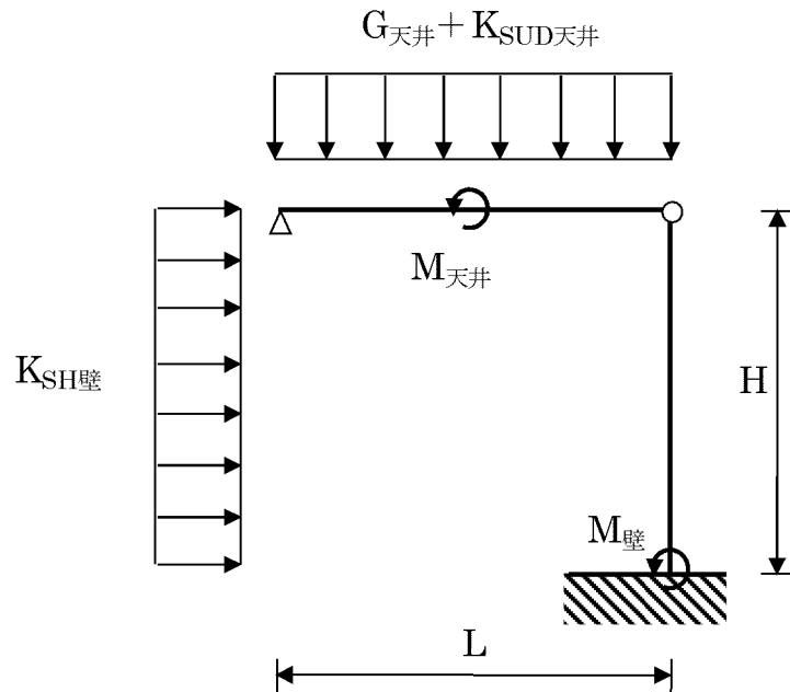
第3-6図 応力模式図 (曲げモーメント)
