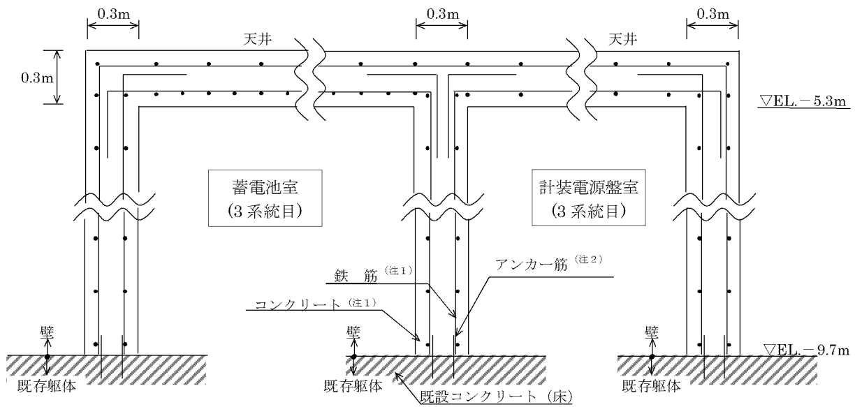
(a) A-A 断面図
