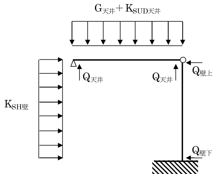
第 3-7 図 応力模式図 (せん断力)
