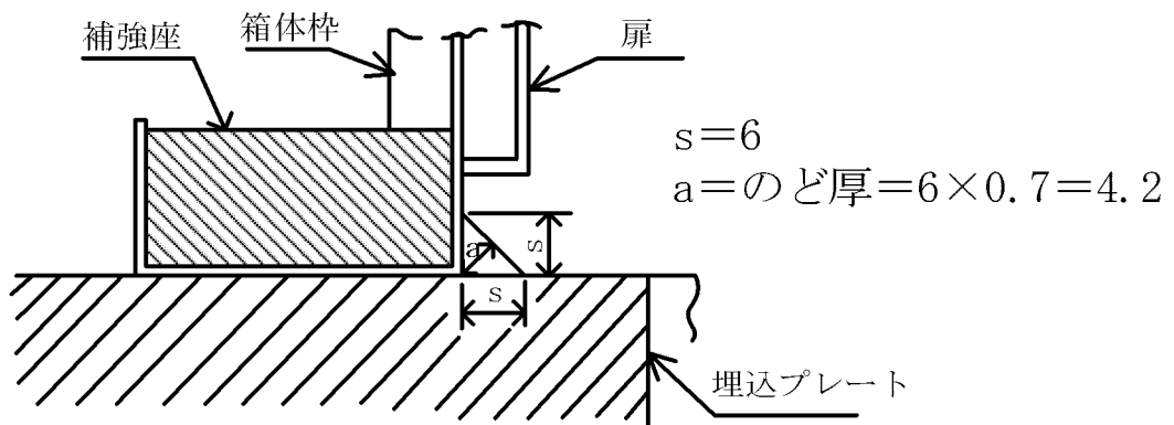
第 5-4 図 溶接サイズ
