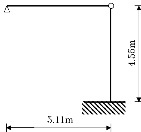
第3-5図 解析モデル
