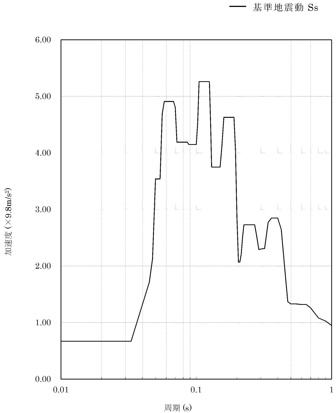
第 5-1 図 (2/2) 基準地震動 (Ss) (原子炉補助建屋EL. 3.7m 減衰定数1.0% 鉛直方向 包絡)
