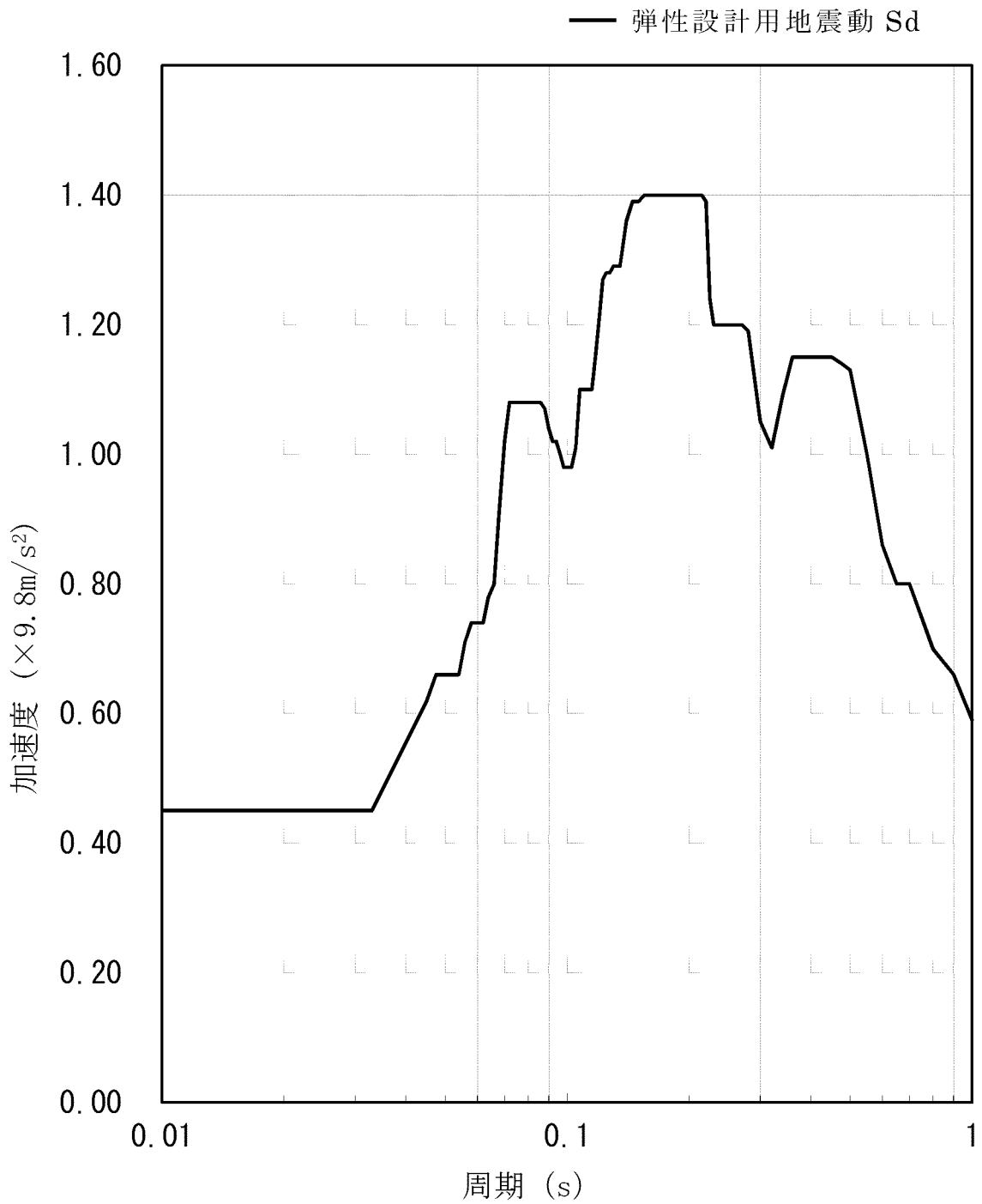
第 5-2 図(1/2) 弾性設計用地震動 Sd (基礎 EL. -10.10m 減衰定数 4.0% 水平方向 包絡)
