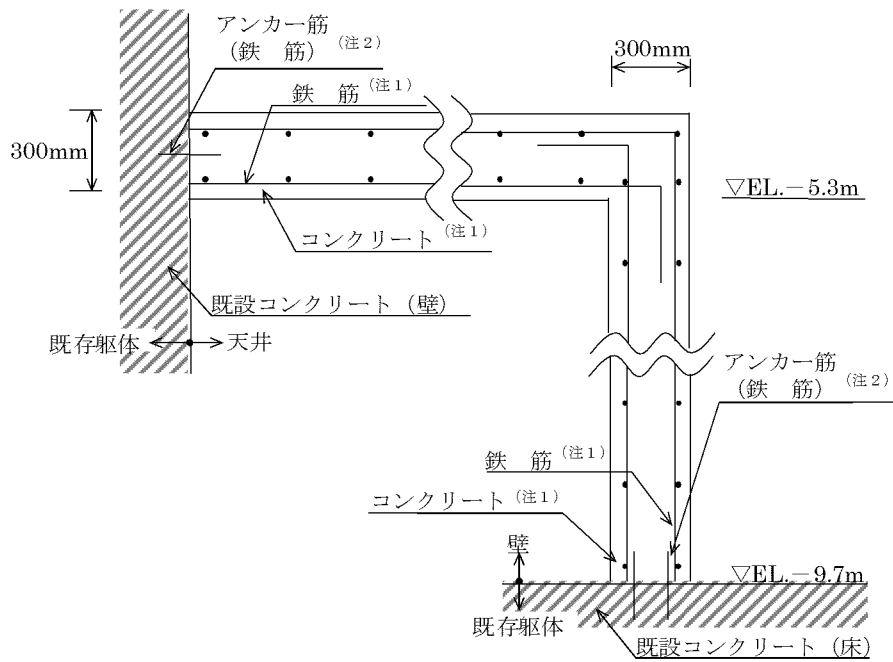
(b) B-B 断面図
