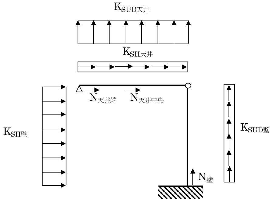
第3-8図 応力模式図(軸力)
