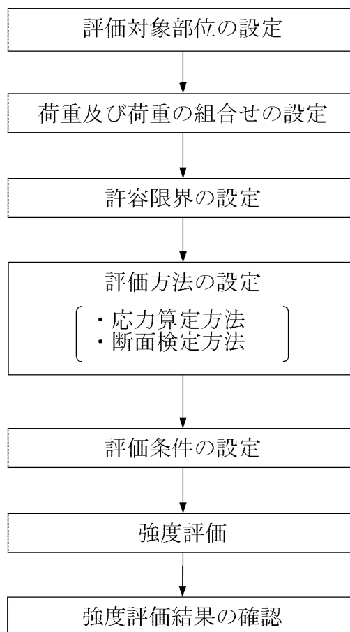
第 2-3 図 4A 原子炉補助建屋堰の強度評価フロー
