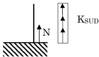
第 4-3 図 4A 原子炉補助建屋堰に生じる応力模式図 (軸力)
