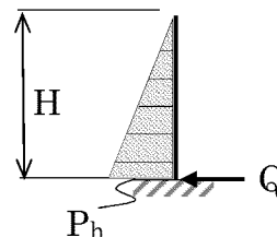
第 3-2 図 4A 原子炉補助建屋堰下端に生じる応力の概念図 (せん断力)
