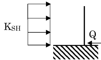
第 4-2 図 4A 原子炉補助建屋堰に生じる応力模式図 (せん断力)
