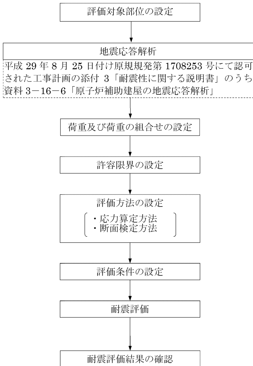
第 2-3 図 4A 原子炉補助建屋堰の耐震評価フロー
