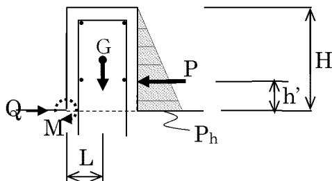
第 4-1 図 4A 原子炉補助建屋堰の 応力算定モデル
