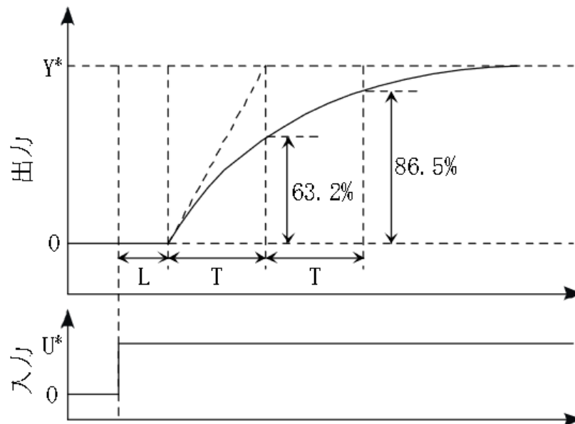
図1 ステップ応答解析
