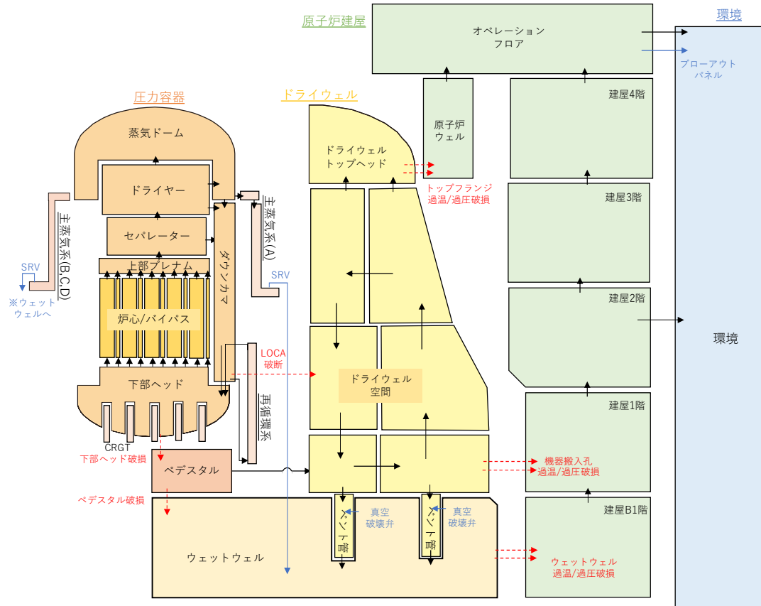
図 1.1 BWR プラントのノード分割及びフローパスの関係図 (イメージ)
