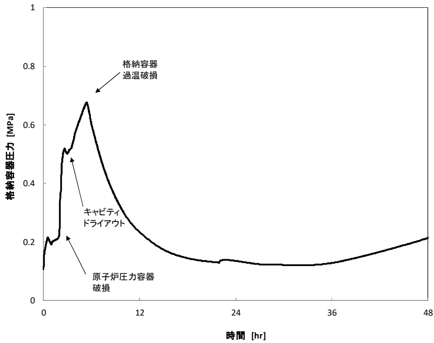
図 1.3 プラント挙動解析結果の整理例
