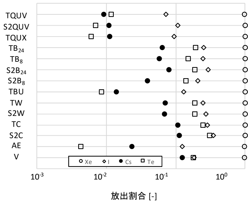
図 1.5 ソースターム解析結果の整理の例
