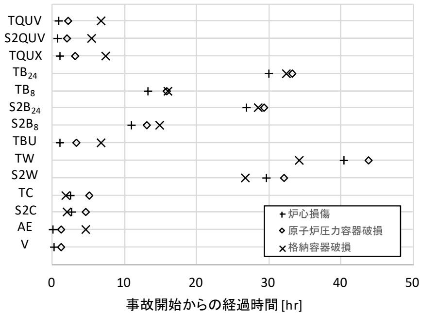
図 1.4 代表シナリオの比較の例
