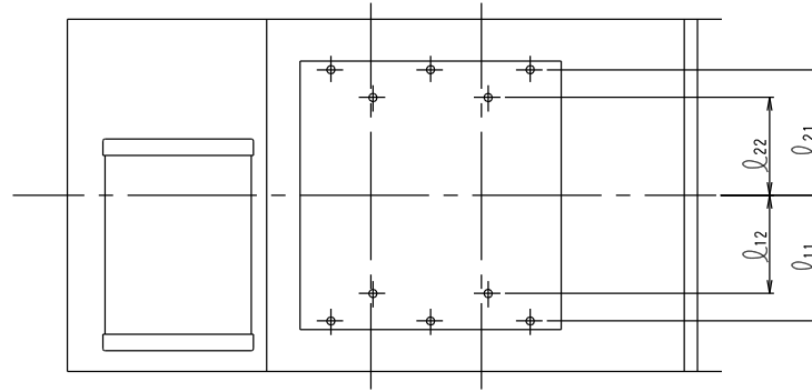
A~A矢視図
