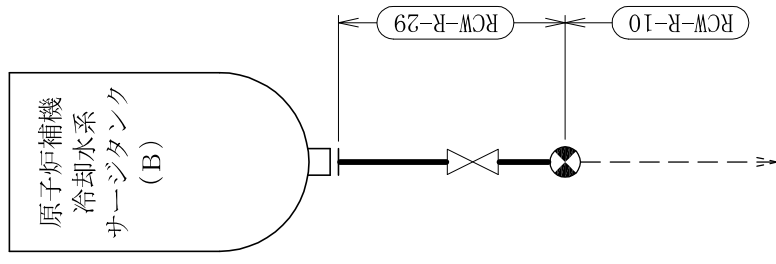
原子炉補機冷却水系概略系統図 (その4) ~
