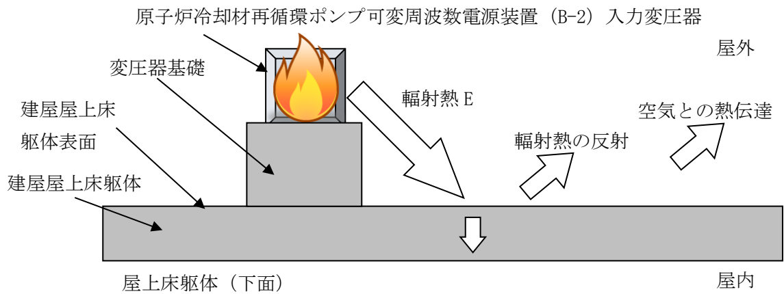
図 2-9 コントロール建屋屋上床躯体表面の計算モデル
