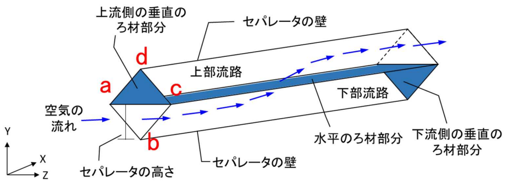
(b) (a)から単位流路を抜き出したもの
