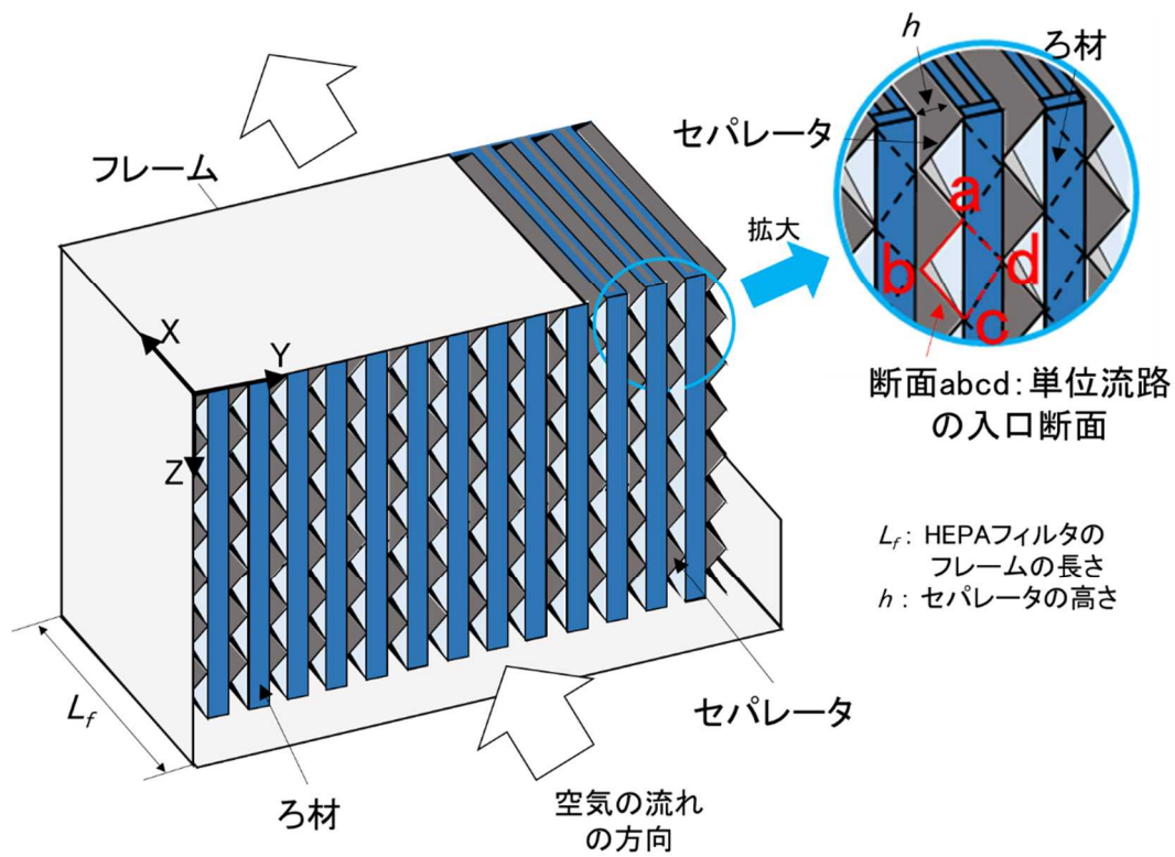
(a) HEPA フィルタの概略図
