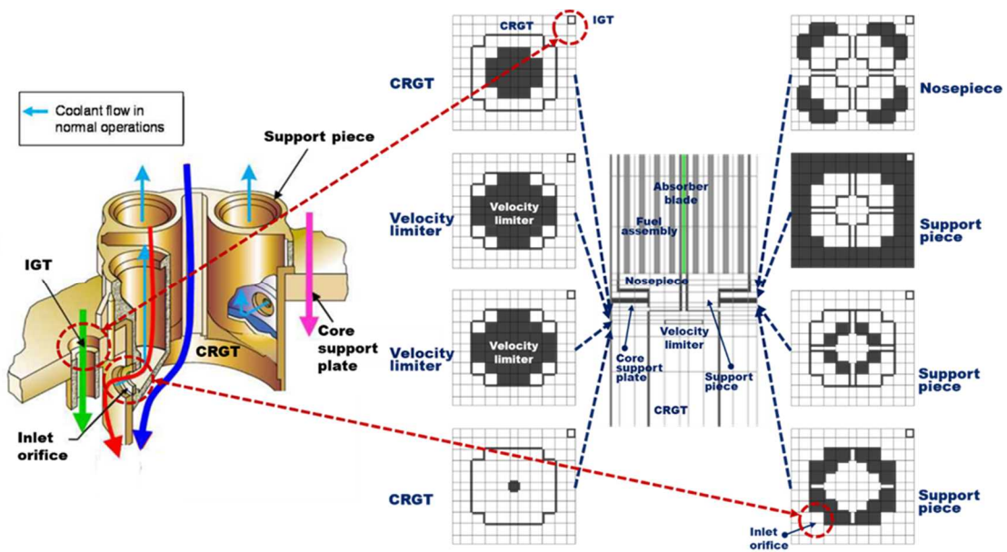
図 1 詳細幾何形状モデルの解析体系
