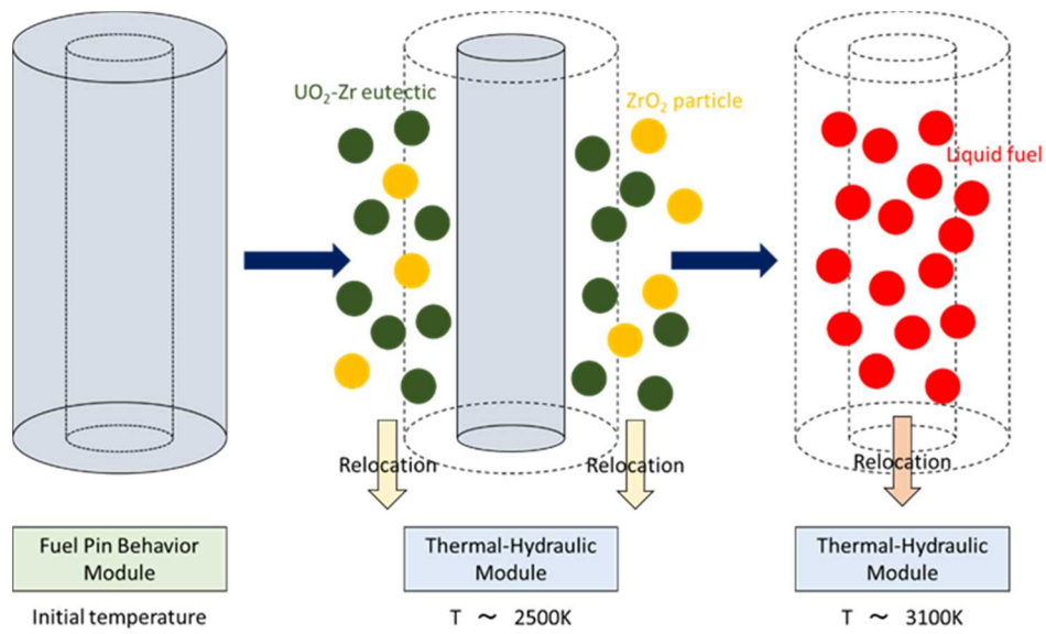
図 2 部分的な燃料破損モデルの概念図
