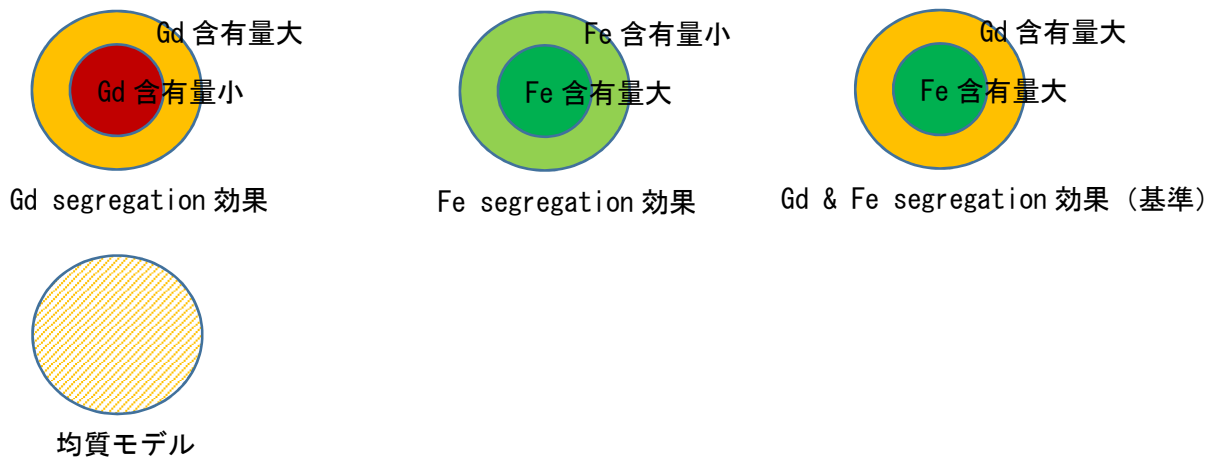
図 4 中性子吸収材の偏在
