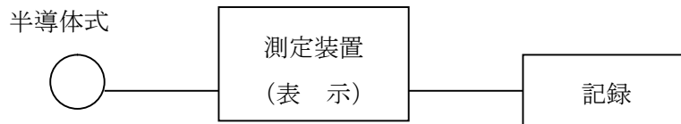
図3-12 可搬型エリアモニタの概略構成図
