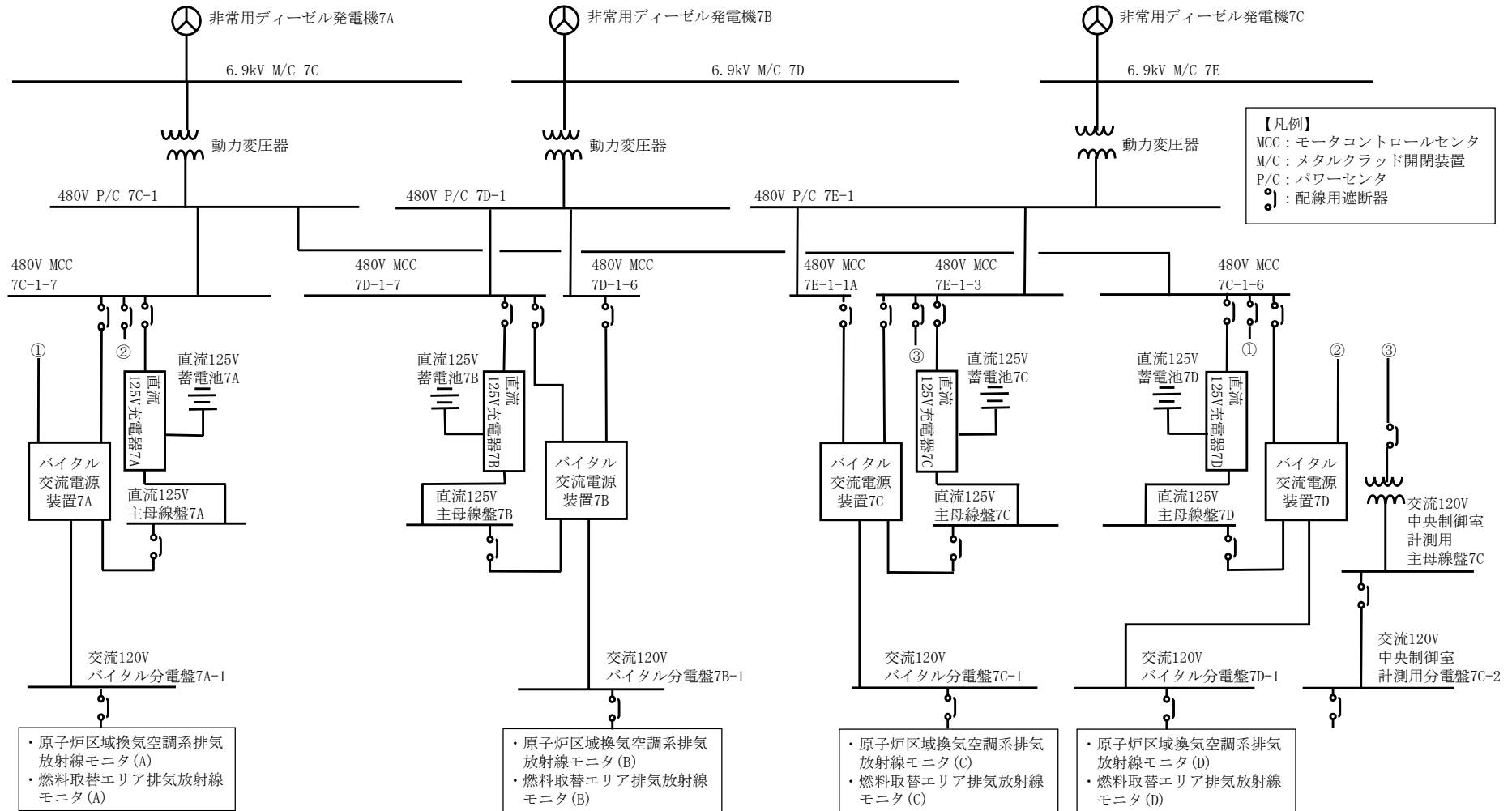
図3-5 燃料取替エリア排気放射線モニタ及び原子炉区域換気空調系排気放射線モニタの概略電源系統図（交流電源）
