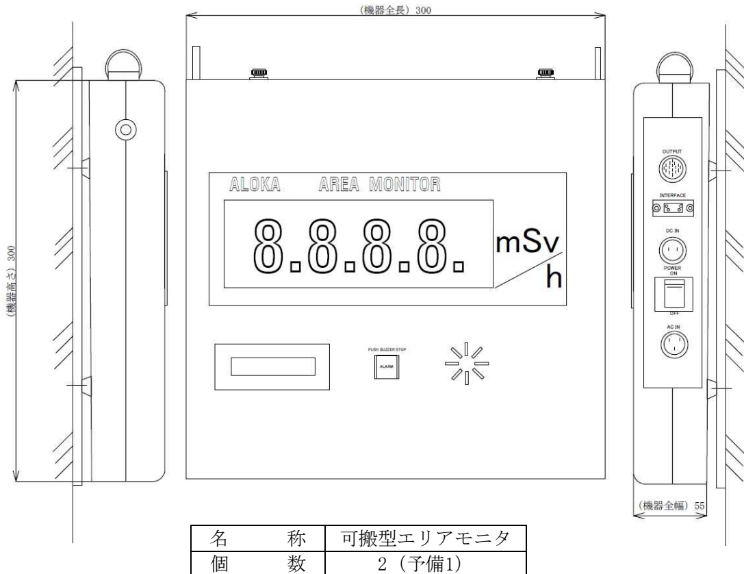
図3-13 検出器の構造図(可搬型エリアモニタ)
