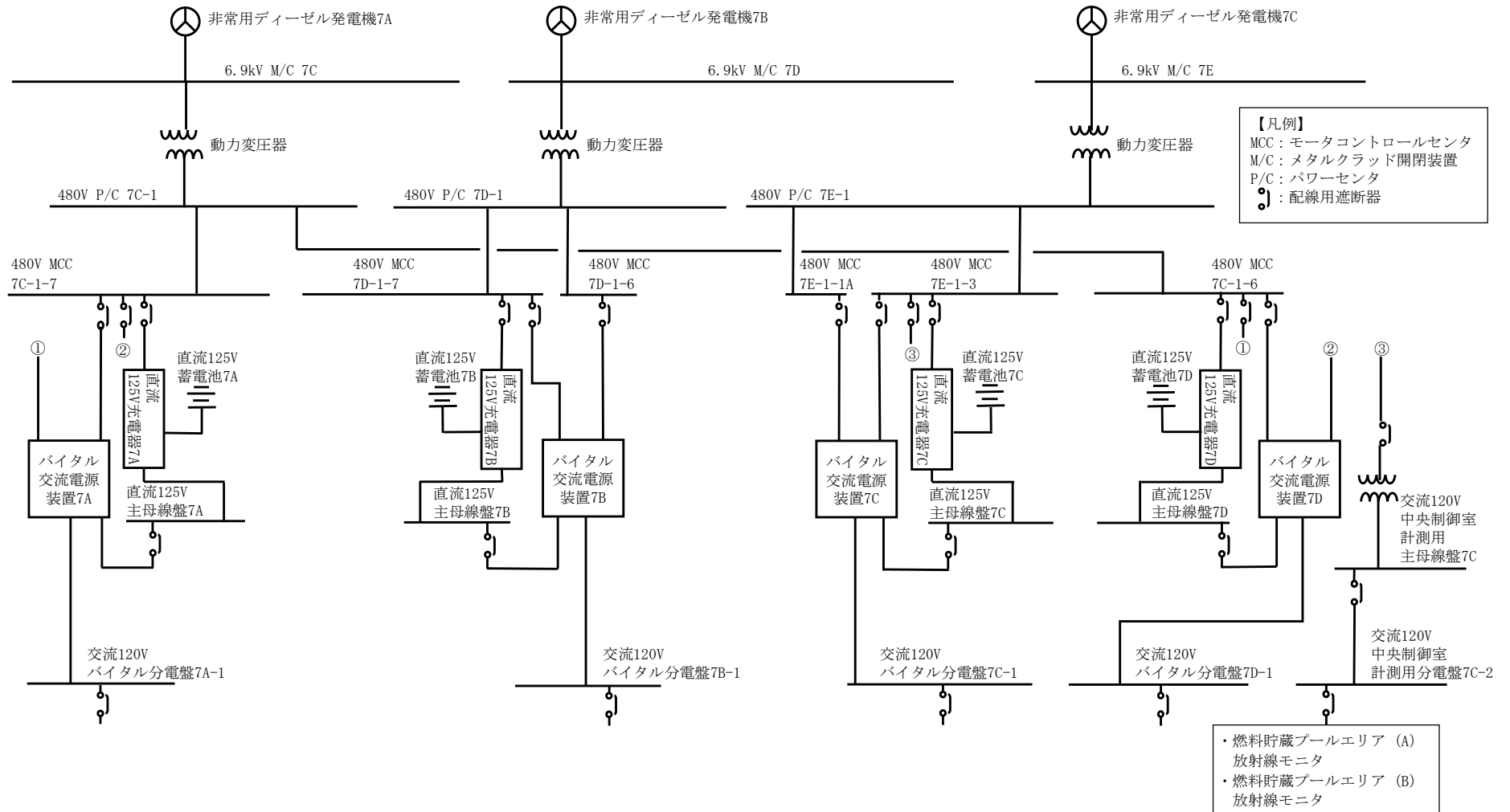
図3-15 燃料貯蔵プールエリア放射線モニタの概略電源系統図（交流電源）
