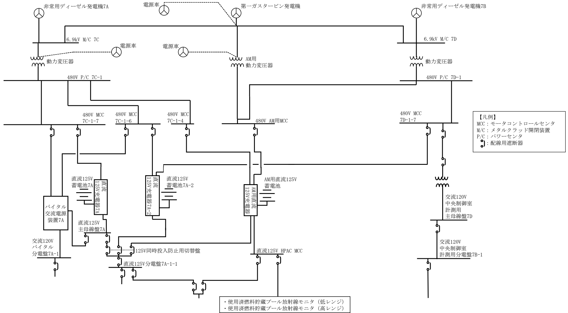
図3-19 使用済燃料貯蔵プール放射線モニタ（低レンジ）（高レンジ）の概略電源系統図（直流電源）
