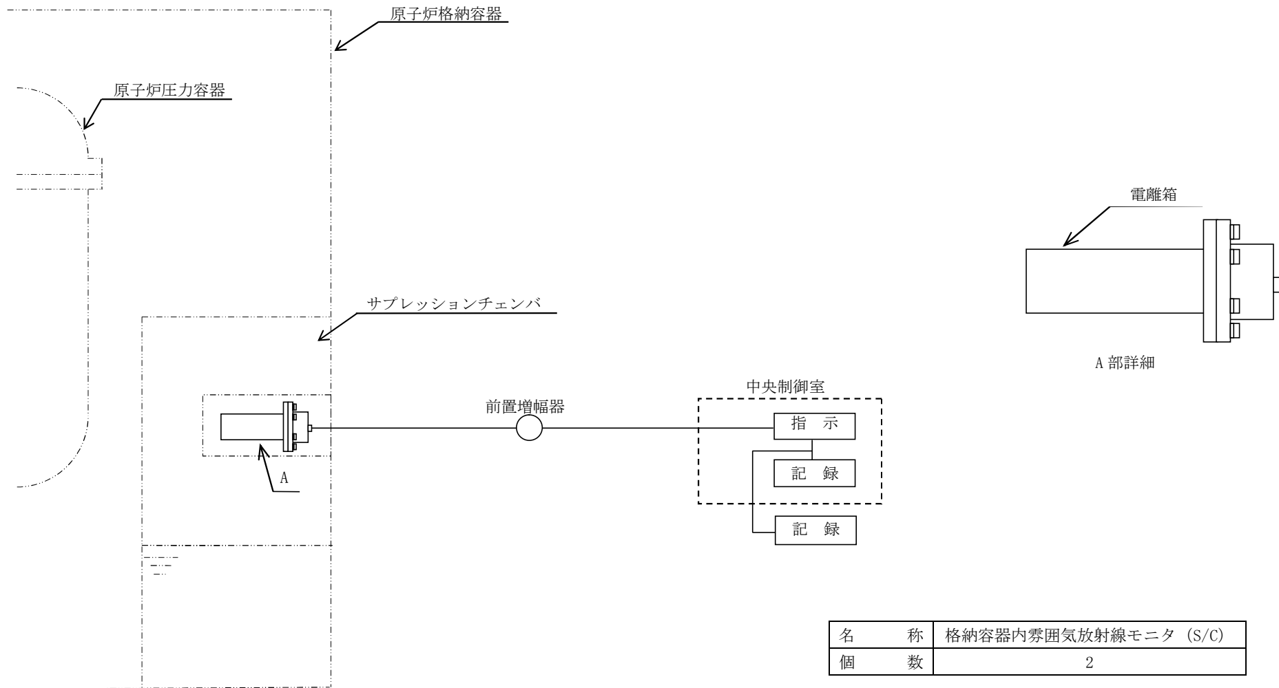
図3-4 検出器の構造図 (格納容器内雰囲気放射線モニタ (S/C) )
