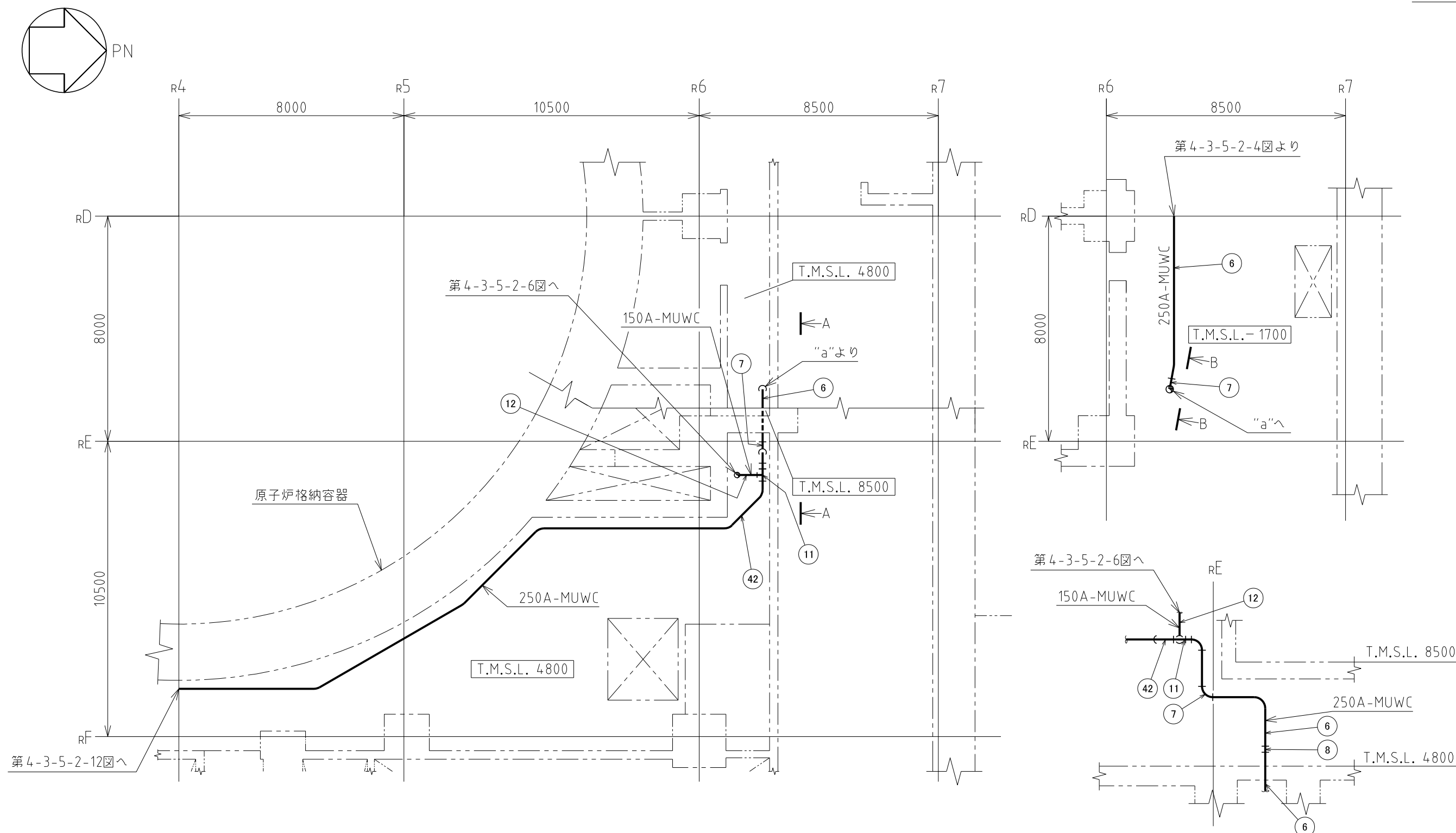
A~A矢視図
