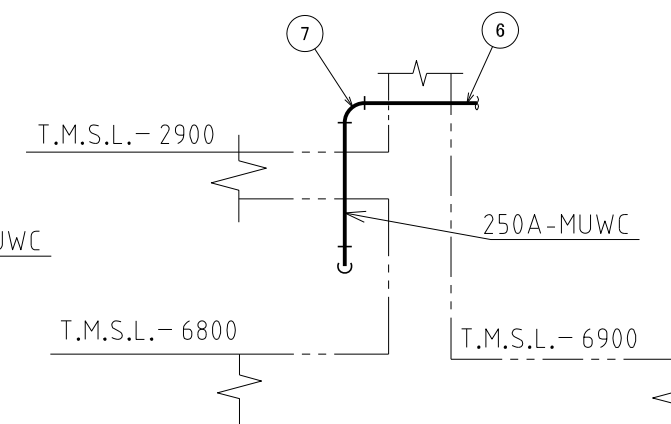
E~E矢視図
