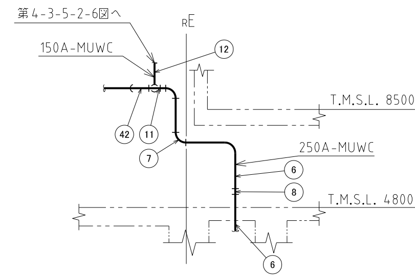
A~A矢視図
