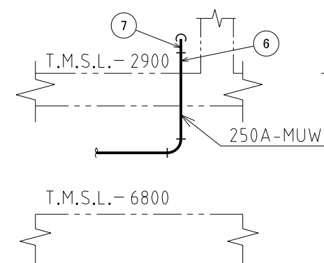
D~D矢視図
