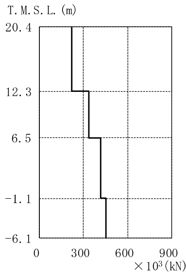
図 4-15 最大応答軸力（基準地震動 S s ，NS 方向，誘発上下動）
