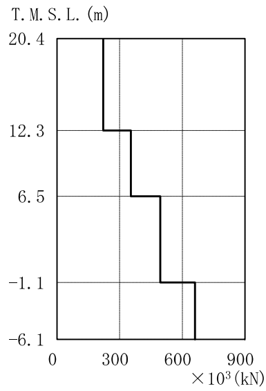
図 4-12 最大応答軸力（基準地震動 S s ，鉛直方向）
