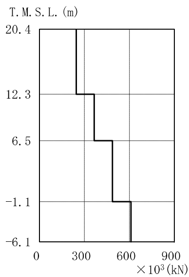
図 4-4 最大応答せん断力（基準地震動 S s , NS 方向）
