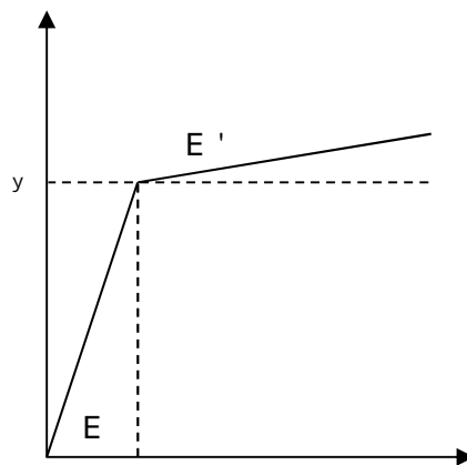
図 3-6 応力 - ひずみ関係の概念図
