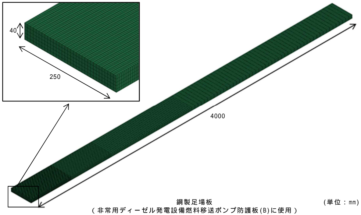
図 3 - 5 飛来物の解析モデル図
