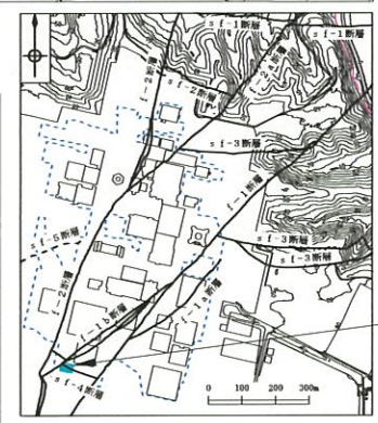
添3-ロ(二)第25図 sf-4断層トレンチ調査スケッチ図
