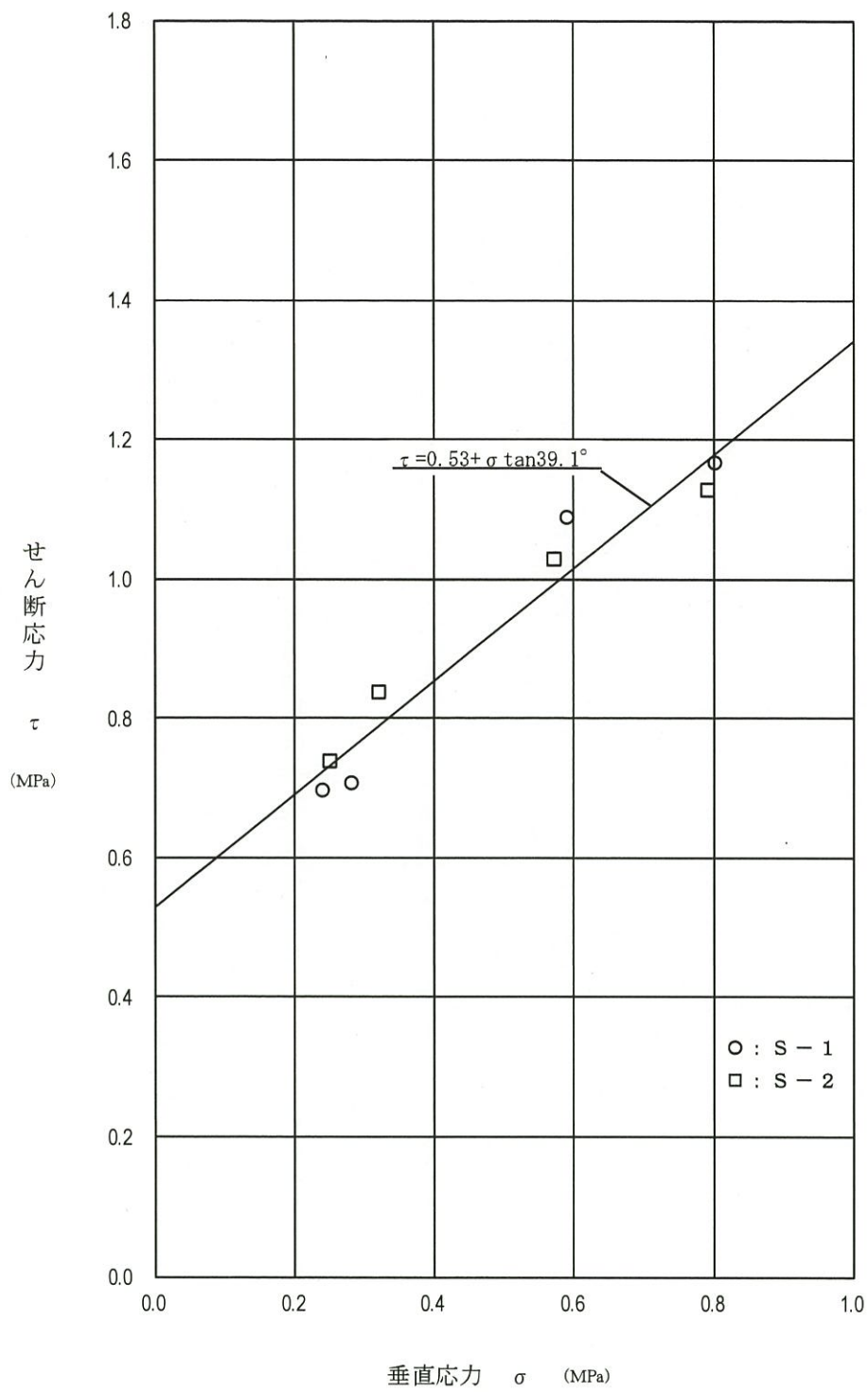
添3-口(二)第32図 岩盤せん断強度及び破壊包絡線
