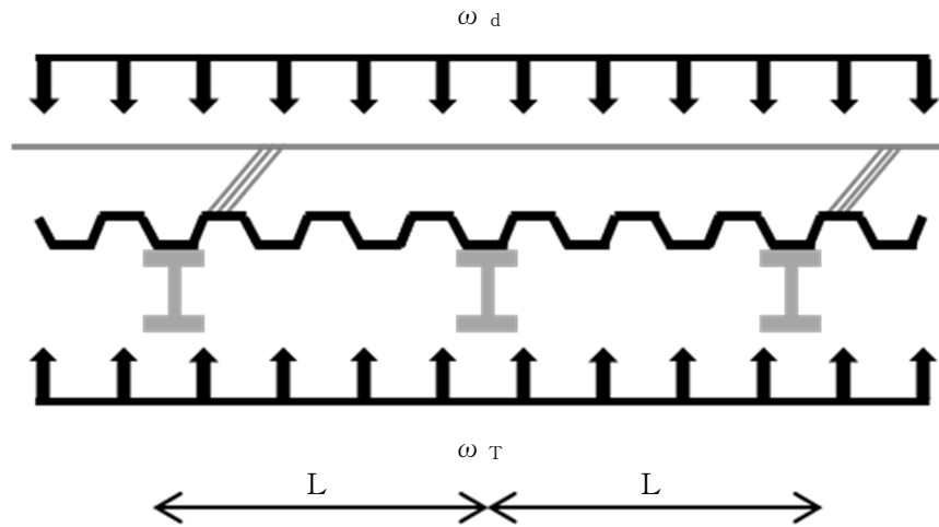
図 3-14 デッキプレートに作用する荷重の概要
