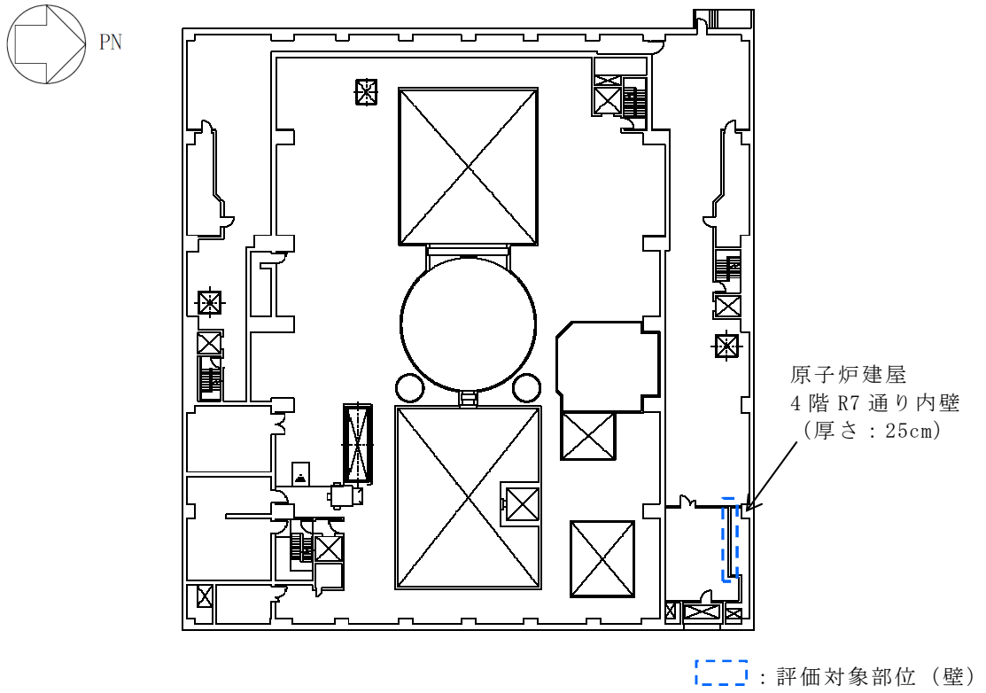
図 2-2 原子炉建屋の概略平面図 (T.M.S.L. 31.7m) (2/2)
