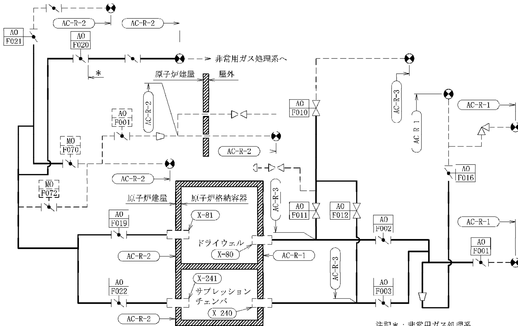
不活性ガス系概略系統図
