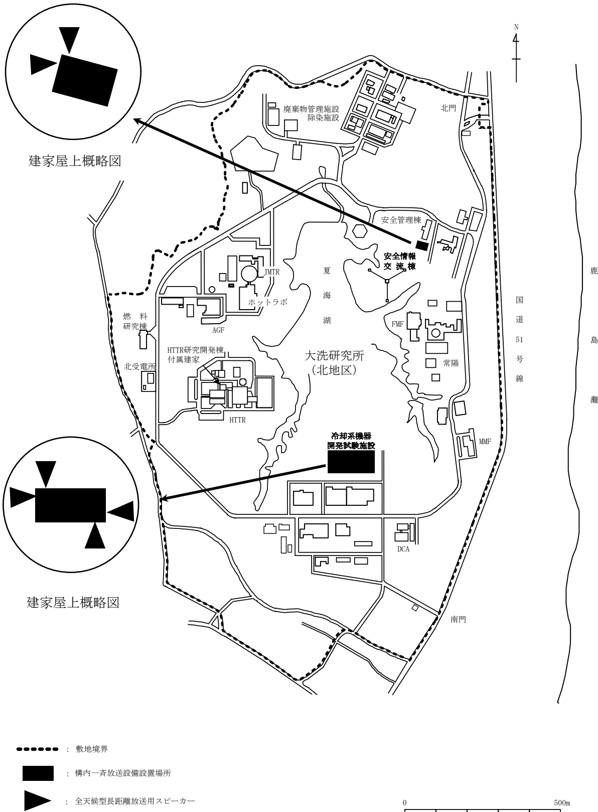
図 3-1 構内一斉放送設備の設置場所
