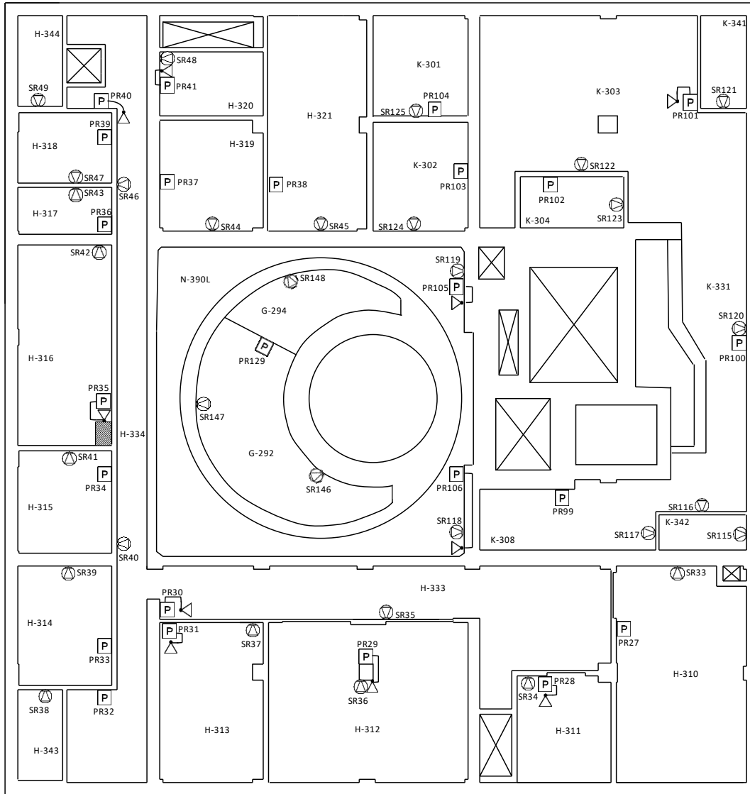
図 3-3-5 非常用放送設備(HTTR)及び送受話器(ページング)の設置場所 (原子炉建家 地下1階)
