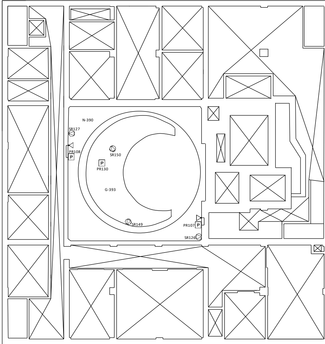
図 3-3-6 非常用放送設備(H T T R)及び送受話器(ページング)の設置場所 (原子炉建家 地下中 1 階)
