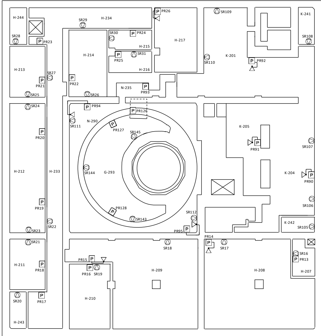
図 3-3-3 非常用放送設備(HTTR)及び送受話器(ページング)の設置場所 (原子炉建家 地下2階(1/2))
