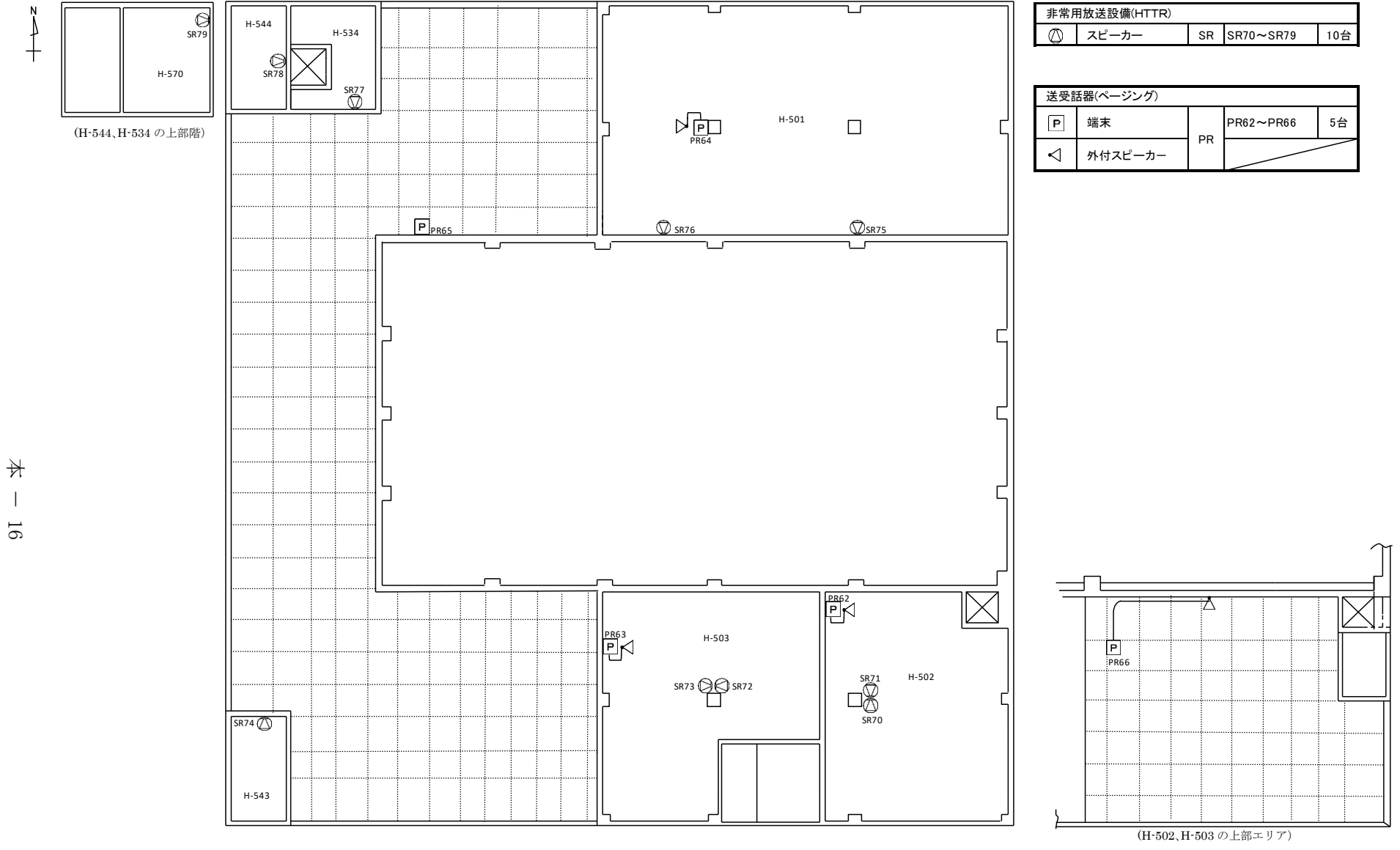
図 3-3-9 非常用放送設備(HTTR)及び送受話器(ページング)の設置場所(原子炉建家 2 階)
