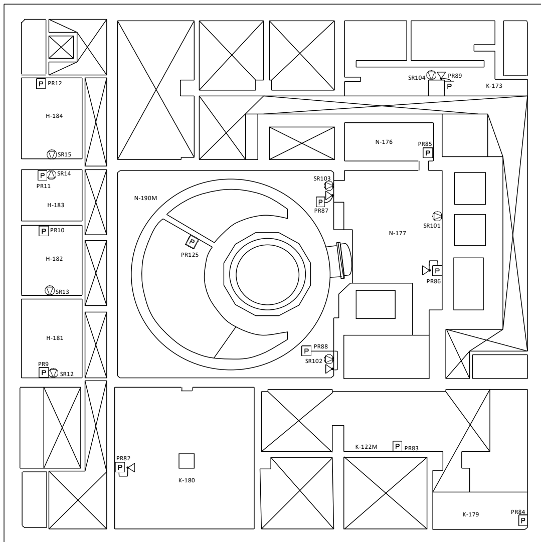
図 3-3-2 非常用放送設備(HTTR)及び送受信器(ページング)の設置場所 (原子炉建家 地下中3階)
