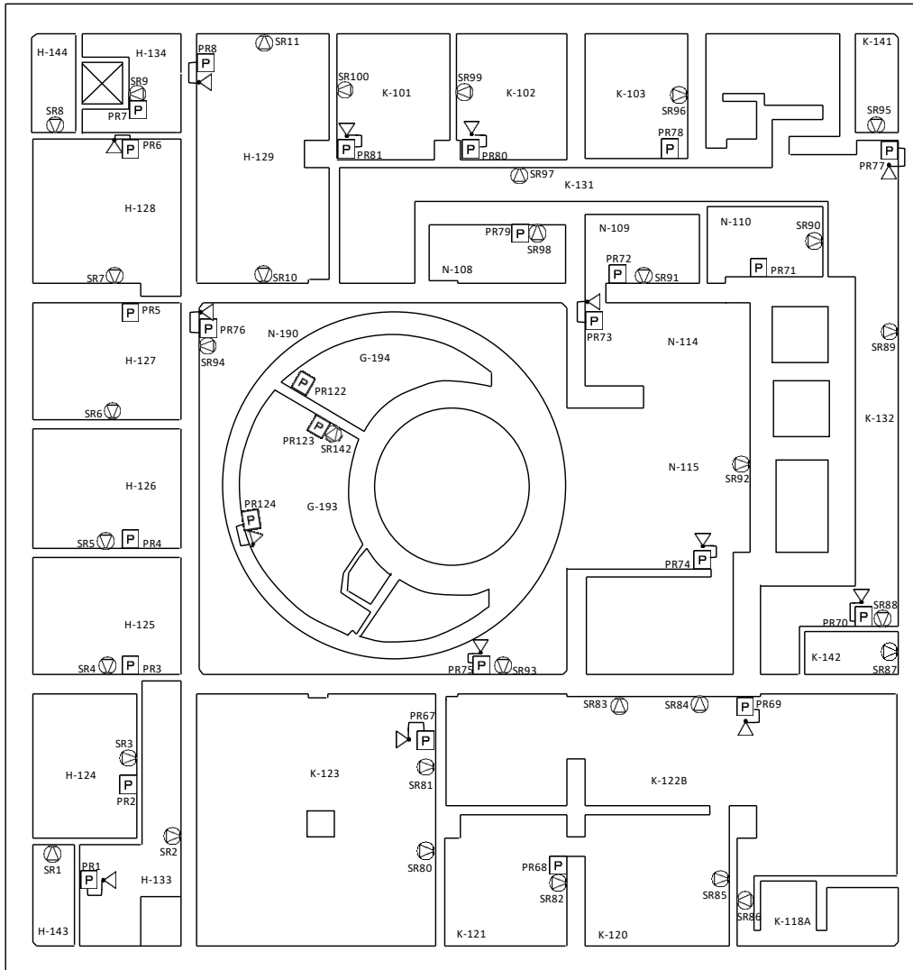
図 3-3-1 非常用放送設備(HTTR)及び送受話器(ページング)の設置場所 (原子炉建家 地下3階)
