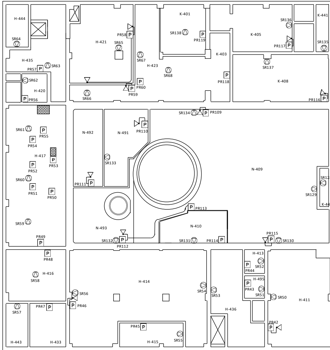
図 3-3-7 非常用放送設備(HTTR)及び送受話器(ページング)の設置場所(原子炉建家 1階(1/2))
