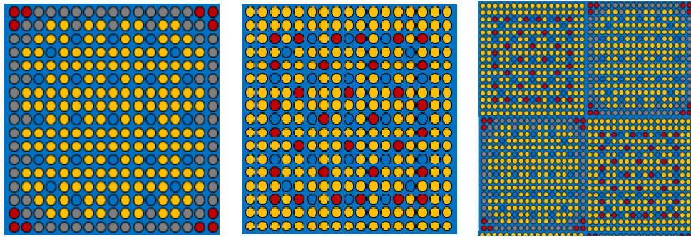
(1) UO 2 燃料集合体単一配置 (2) MOX 燃料集合体単一配置 (3) UO 2 /MOX 燃料集合体市松配置
