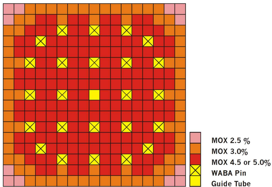
図 5 MOX ベンチマーク問題の MOX/UO 2 燃料集合体の燃料棒配置
