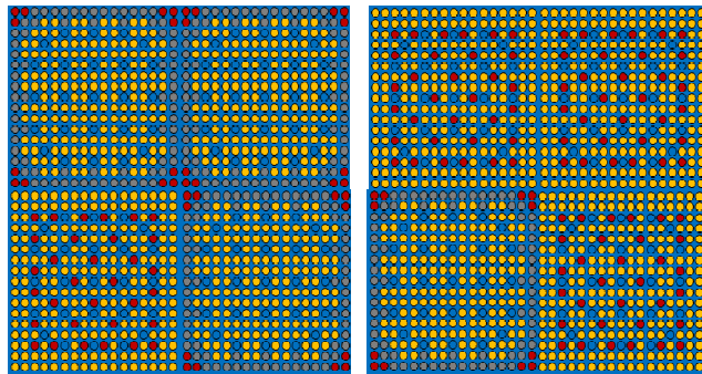
(4) 1/3MOX 相当の燃料集合体配置 (5) 2/3MOX 相当の燃料集合体配置
