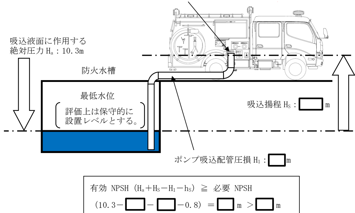
図3-3 可搬型代替注水ポンプ (A-2級) の有効 NPSH 評価の概略図
