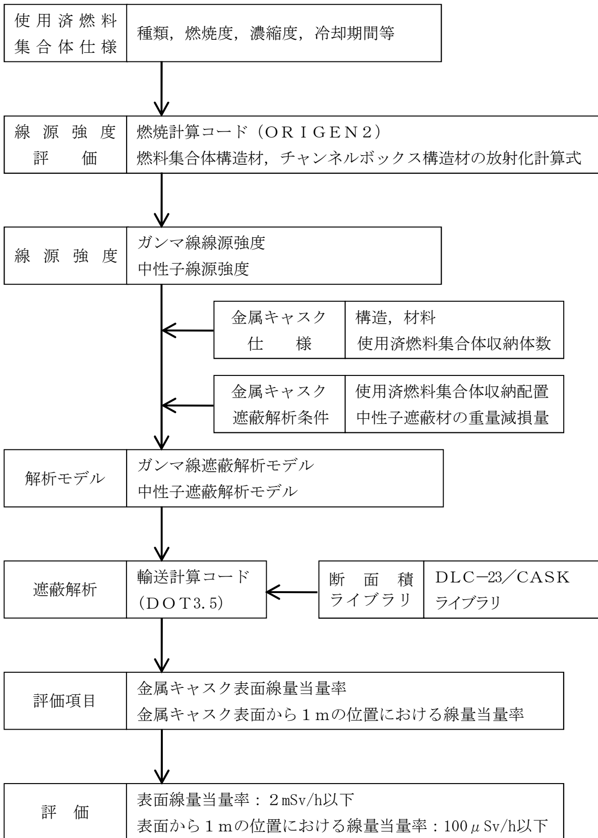
第3.3-2図 金属カスクの遮蔽解析フロー
