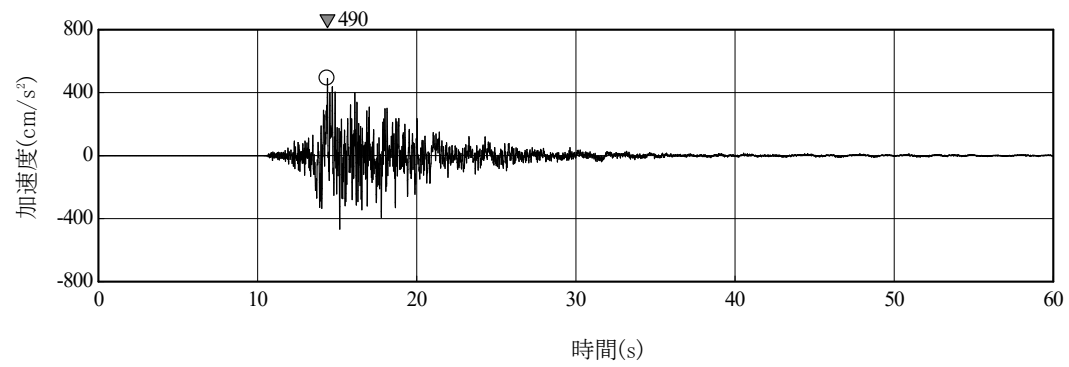
(b) 基準地震動 Ss-B2H2 (水平方向)
