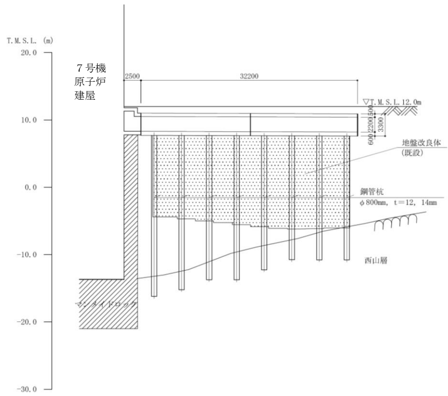
図 2-4 燃料移送系配管ダクトの縦断図 (C-C断面)
