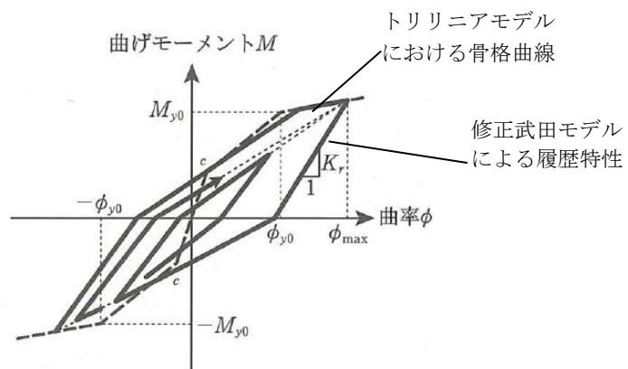
図 3-5 鉄筋コンクリート部材の履歴特性
