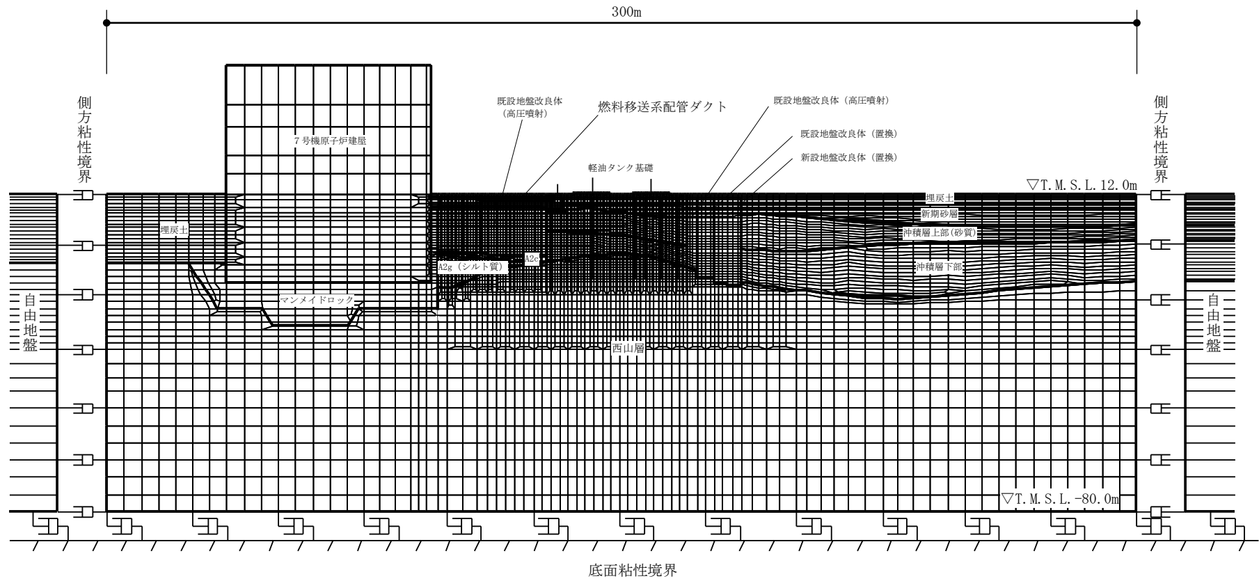
図 3-11 (3) 燃料移送系配管ダクトの地震応答解析モデル (C-C断面 機器・配管系に対する加速度応答抽出用)
