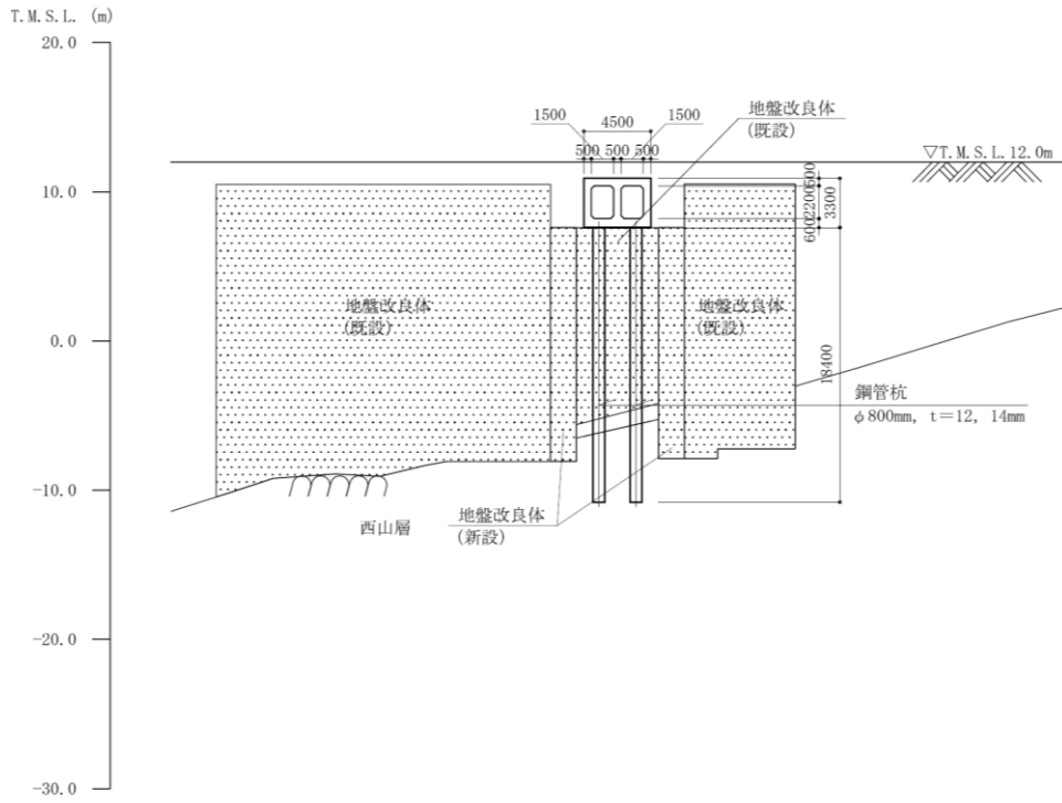
図 2-3(2) 燃料移送系配管ダクトの断面図（B-B断面）
