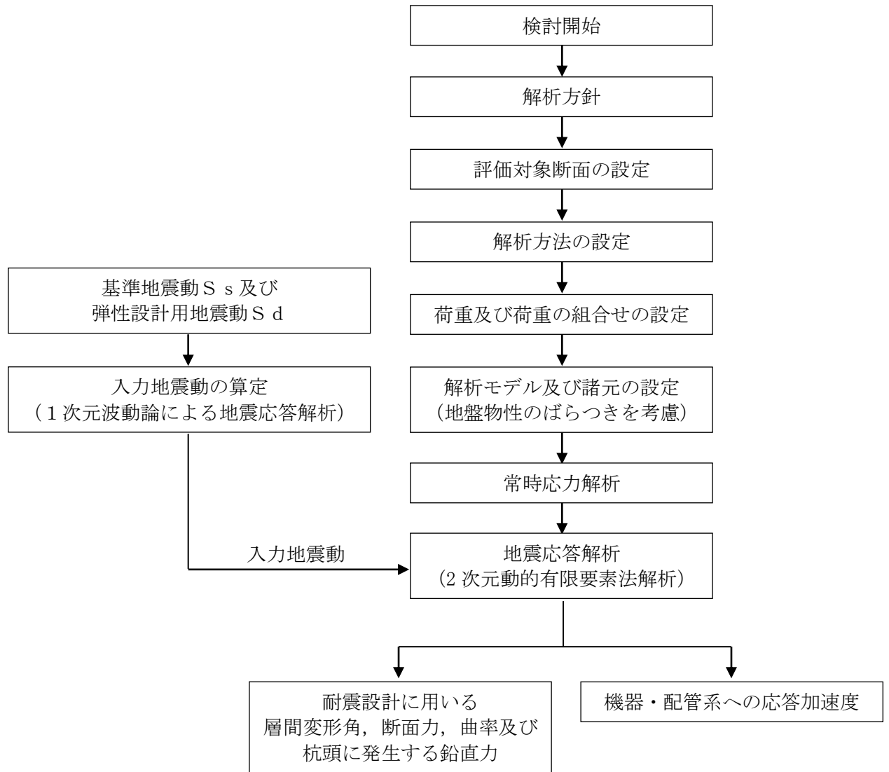
図 2-5 燃料移送系配管ダクトの地震応答解析フロー
