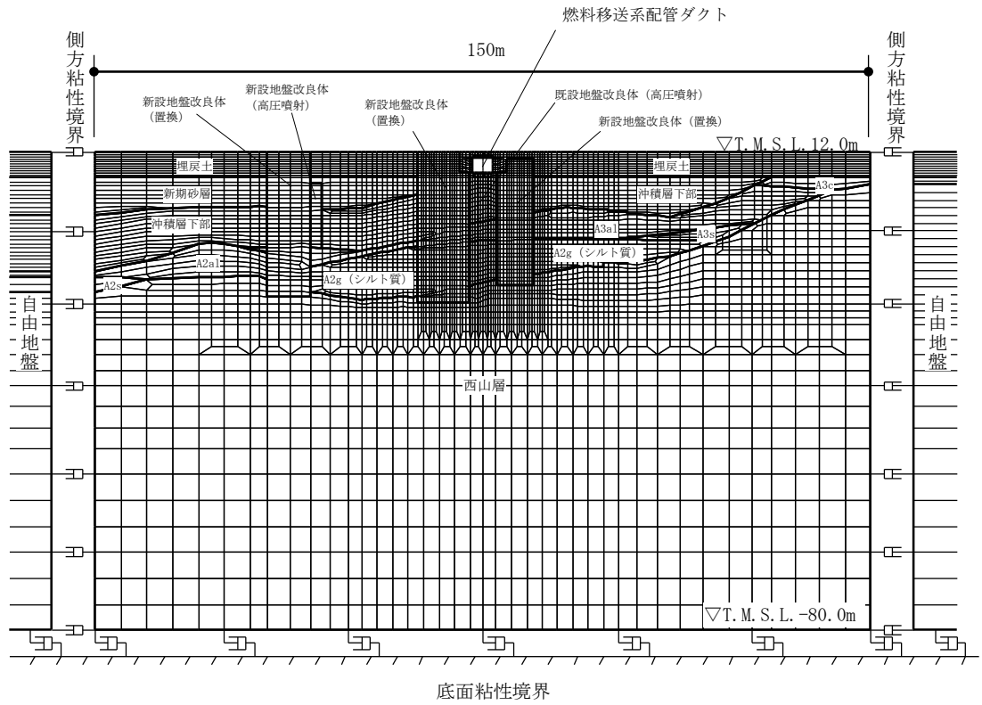
図 3-11 (1) 燃料移送系配管ダクトの地震応答解析モデル (A-A断面)
