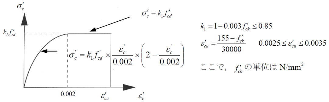
図 3-4(1) 構造部材の非線形特性（コンクリートの応力-ひずみ関係） （原子力発電所屋外重要構造物の耐震性能照査指針・マニュアル（土木学会，2005年）より引用）
