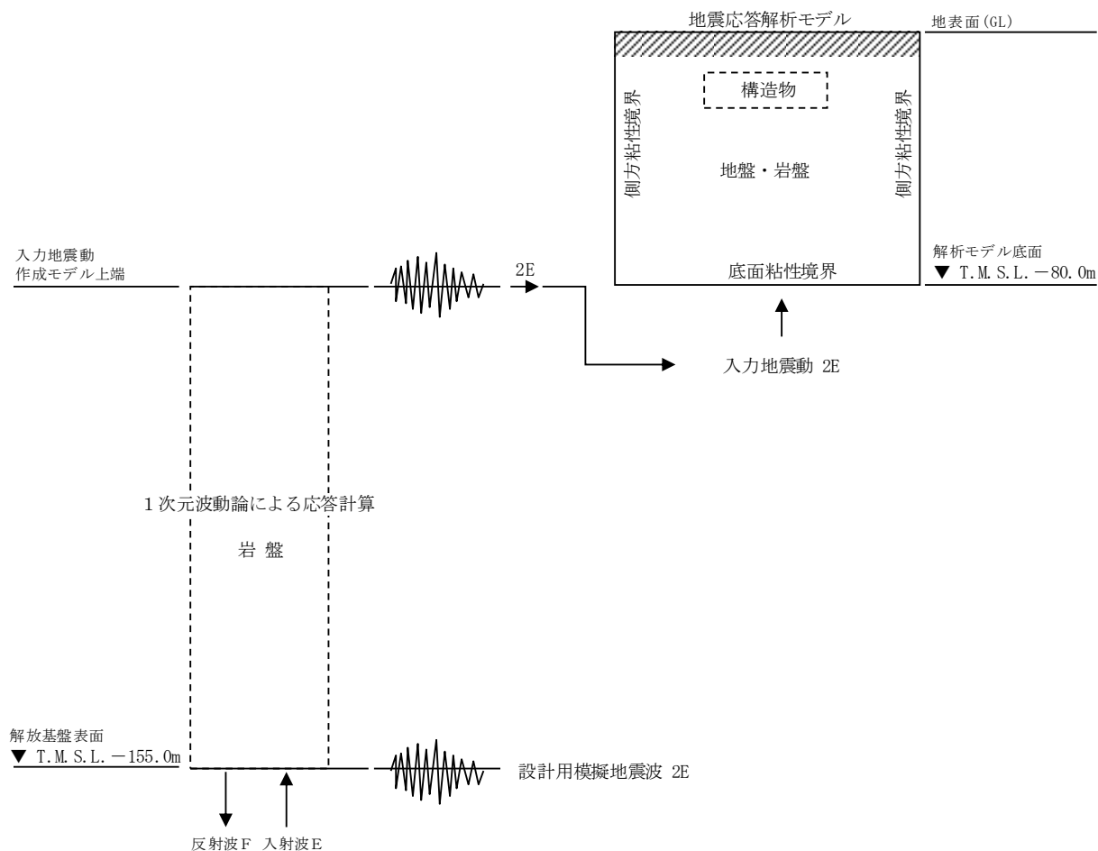
図 3-8 入力地震動算定の概念図
