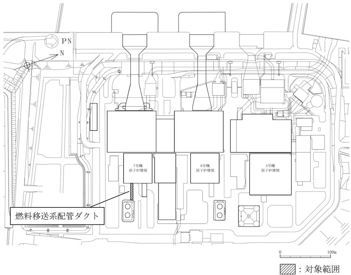
図 2-1 燃料移送系配管ダクトの位置図
