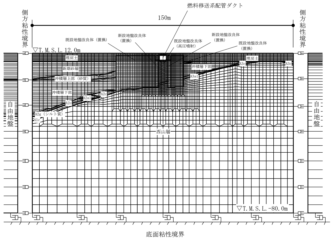
図 3-11 (2) 燃料移送系配管ダクトの地震応答解析モデル (B-B断面)
