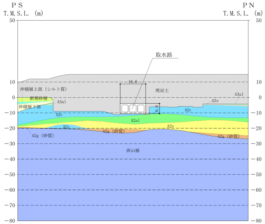
図 3-2 (2) 取水路の評価対象断面図 (B-B断面)
