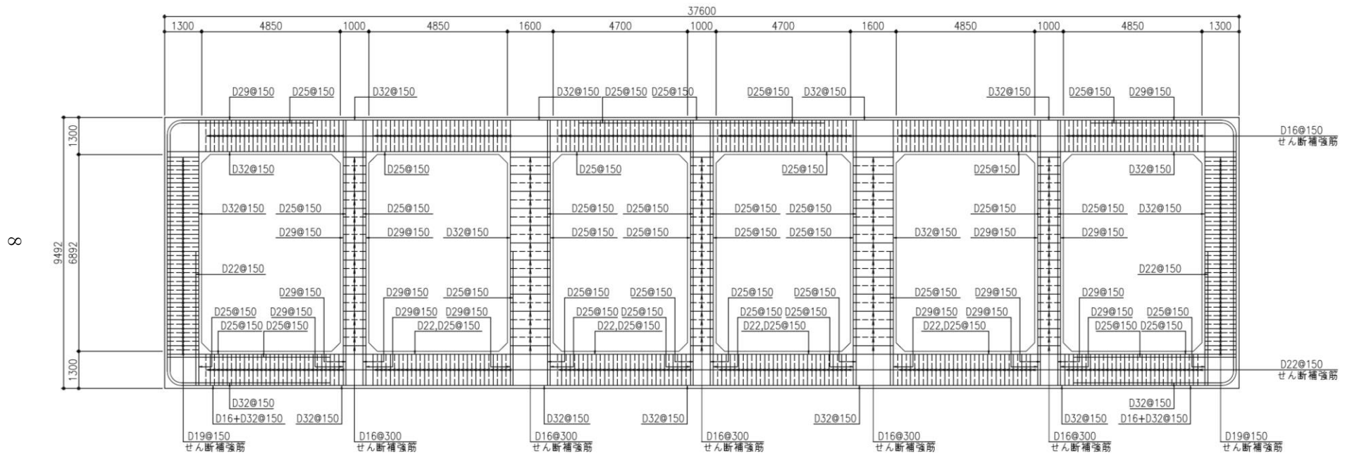
(C-C断面)
