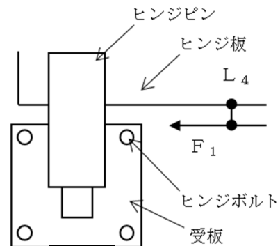
図 4-5 ヒンジピンに生じる荷重の例
