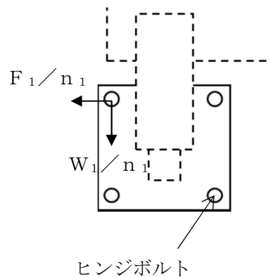
図 4-6 ヒンジボルトに生じる荷重の例
