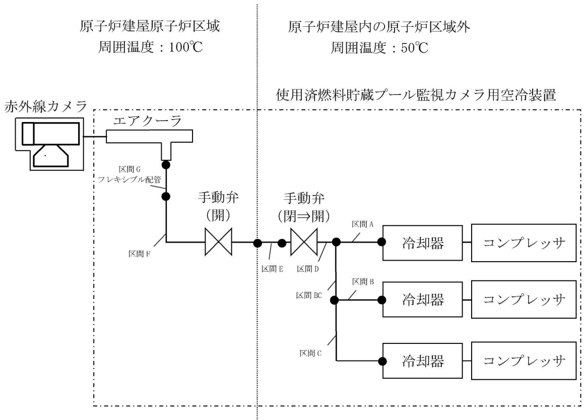
図 1 使用済燃料貯蔵プール監視カメラ用空冷装置の空気供給概略図
