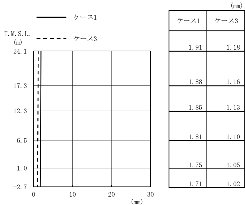
図4-22 最大応答変位 (Ss-1, NS方向, 誘発上下動)
