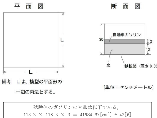
第1図 10型粉末消火器（油火災の消火能力単位：7）の試験体
