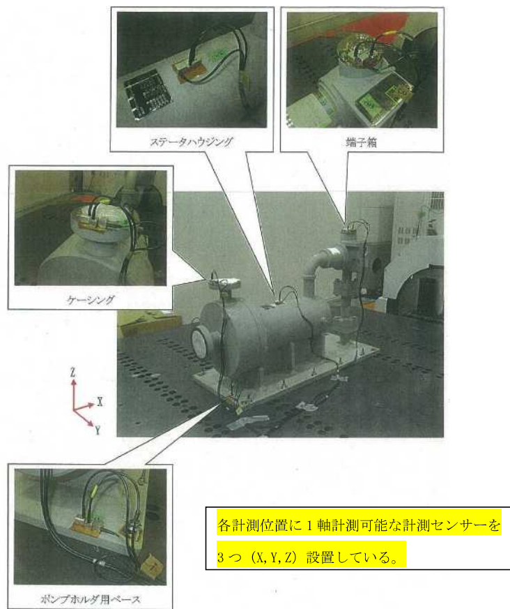
図 2-2 計測センサー取付位置 (その 2)
