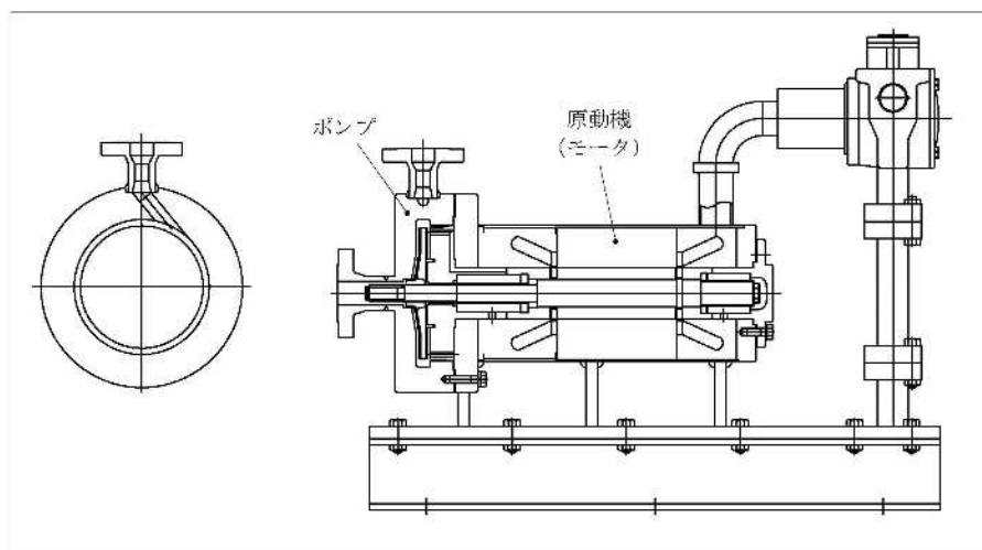
図 1-1 ドレン移送ポンプ断面図
