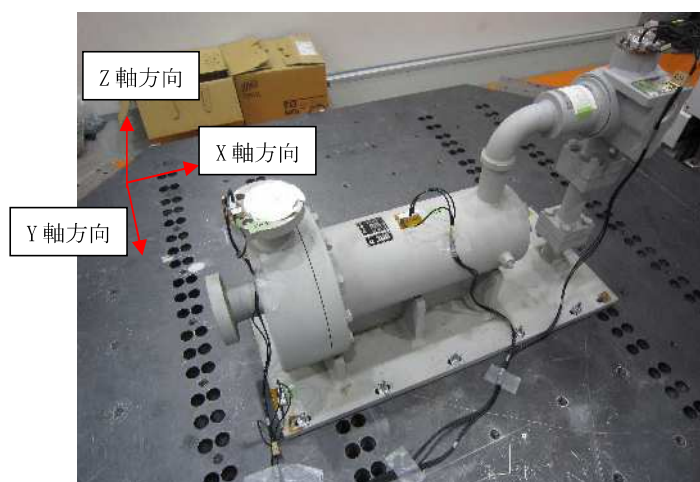
図 1-2 振動試験装置外観
