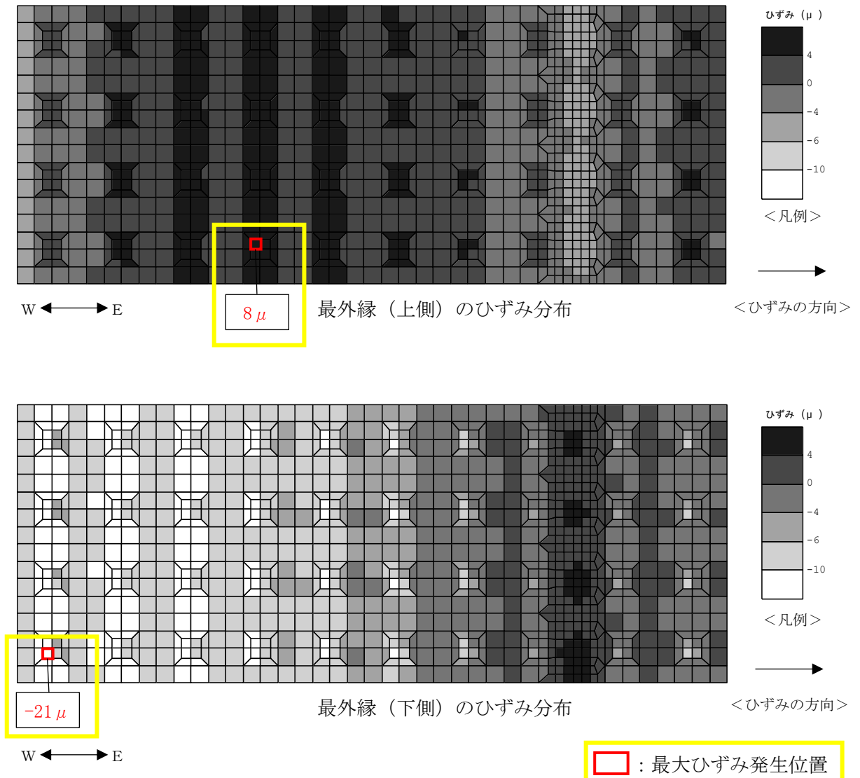
図 6-1 鉄筋コンクリート部材の曲げ軸力照査が最も厳しくなるケースでのひずみ分布図 (第一ガスタービン発電機基礎, 解析ケース①, 地震動 Ss-1+-, t=5.93s)
