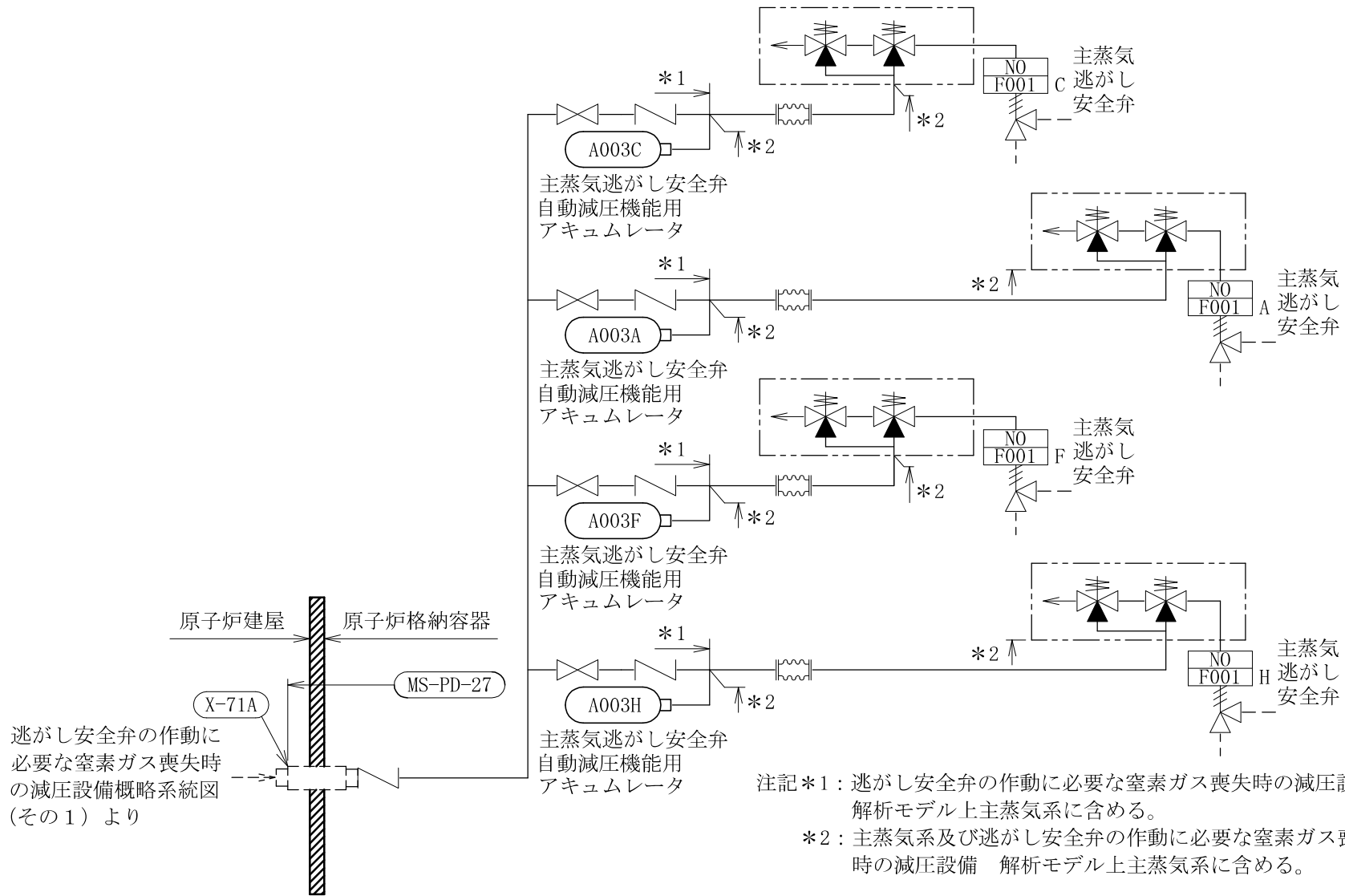
逃がし安全弁の作動に必要な窒素ガス喪失時の減圧設備概略系統図 (その3)
