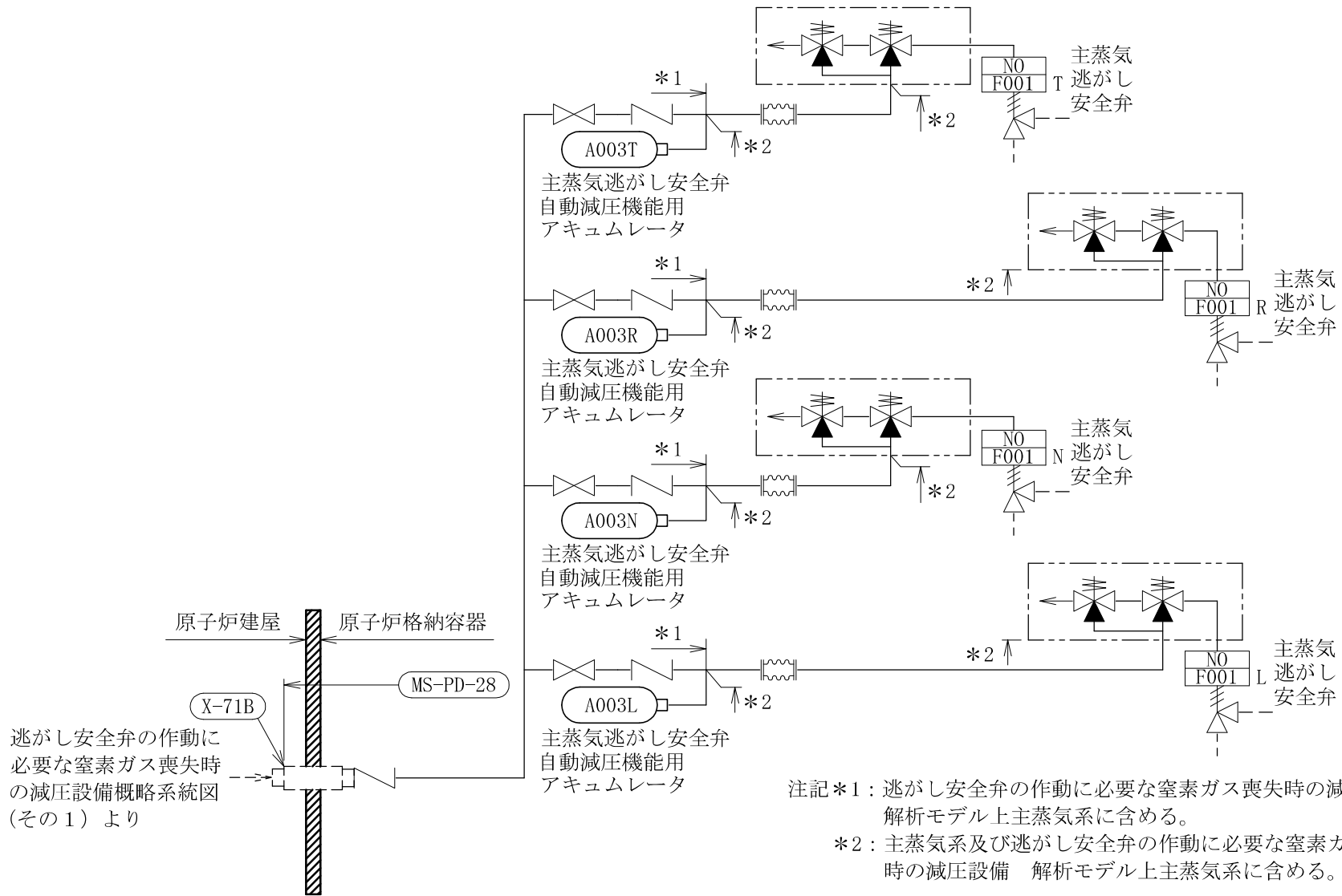
逃がし安全弁の作動に必要な窒素ガス喪失時の減圧設備概略系統図 (その5)
