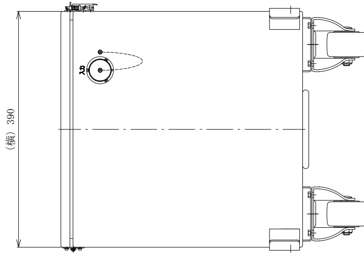
正面図
