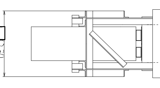
側面図
