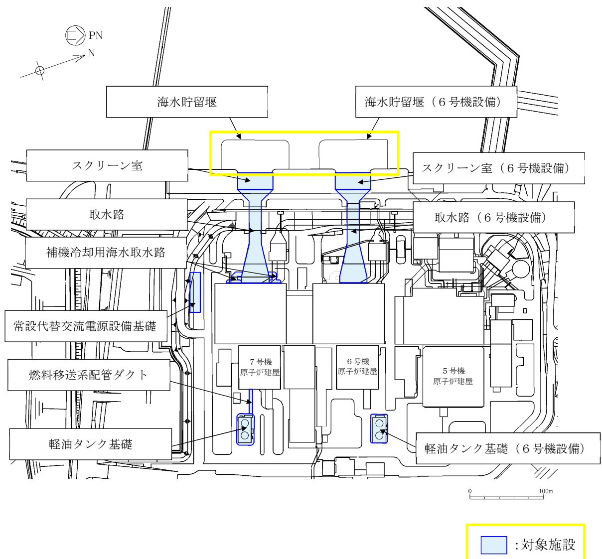
図 1-1 屋外重要土木構造物等位置図
