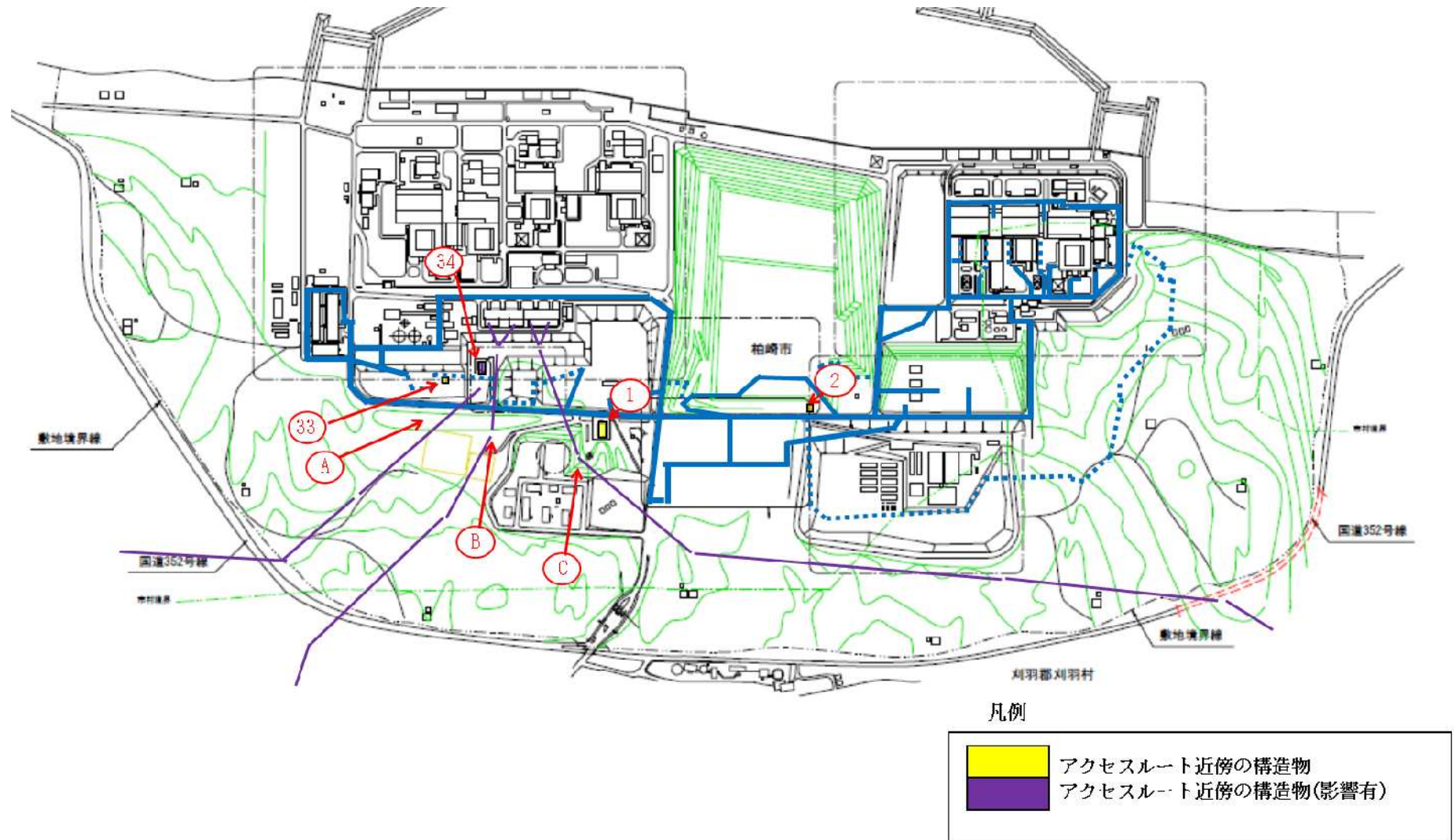
図 7-14 建屋倒壊時の屋外アクセスルートへの影響評価結果（発電所全体図）
