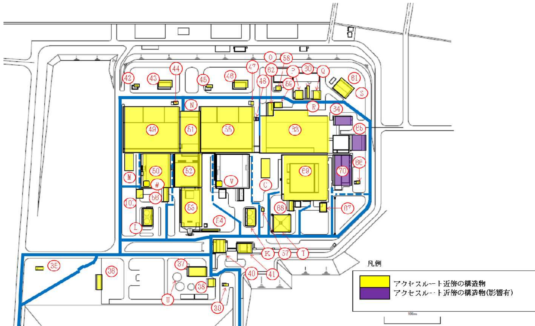
図 7-16 建屋倒壊時の屋外アクセスルートへの影響評価結果（大湊側詳細図）
