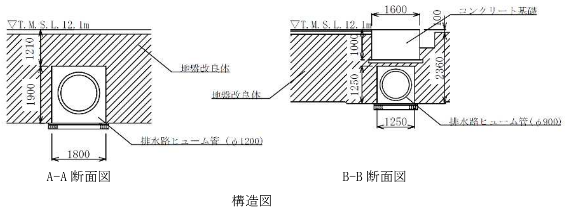
図5-10 保管場所を横断する地中埋設構造物位置及び構造図 (5号機東側第二保管場所)
