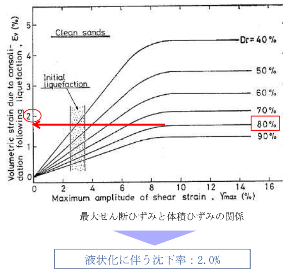
図4-5 Ishihara ほか(1992)の地盤の相対密度に応じた最大せん断ひずみと体積ひずみの関係及び想定する沈下率
