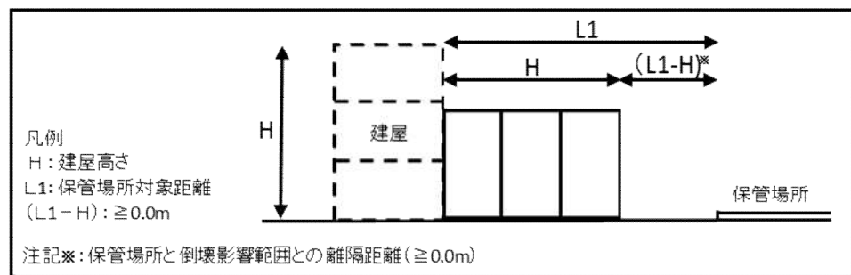
図 7-10 保管場所と倒壊影響範囲との離隔距離の設定方針
