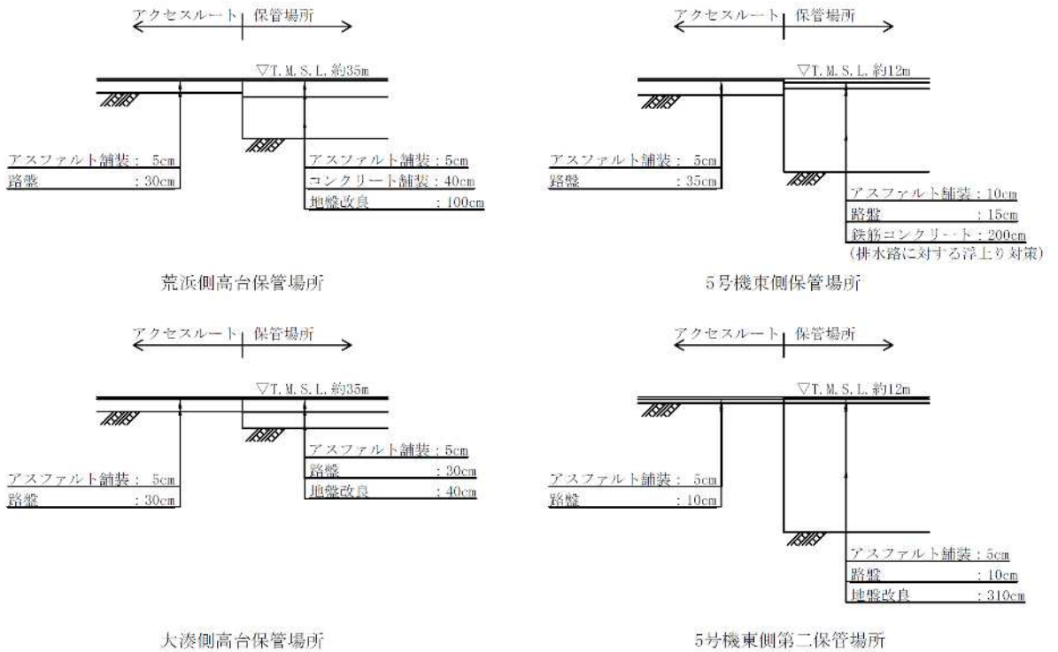
図 5-1 液状化及び揺すり込みによる不等沈下に対する影響評価位置図及び断面図
