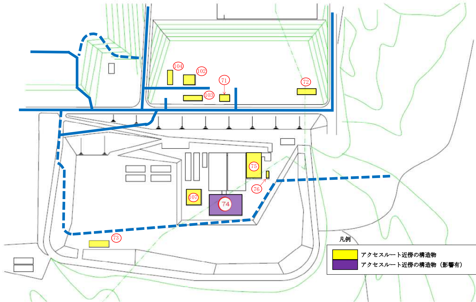
図 7-17 建屋倒壊時の屋外アクセラートへの影響評価結果 (大湊側高台詳細図)
