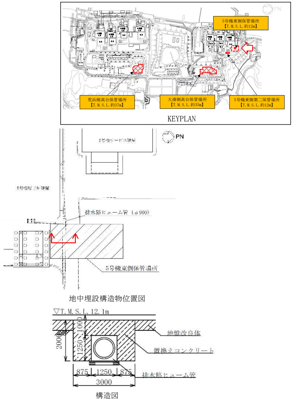
図5-9 保管場所を横断する地中埋設構造物位置及び構造図 (5号機東側保管場所)
