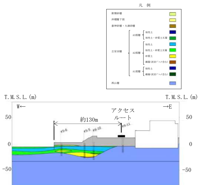
地質断面図
