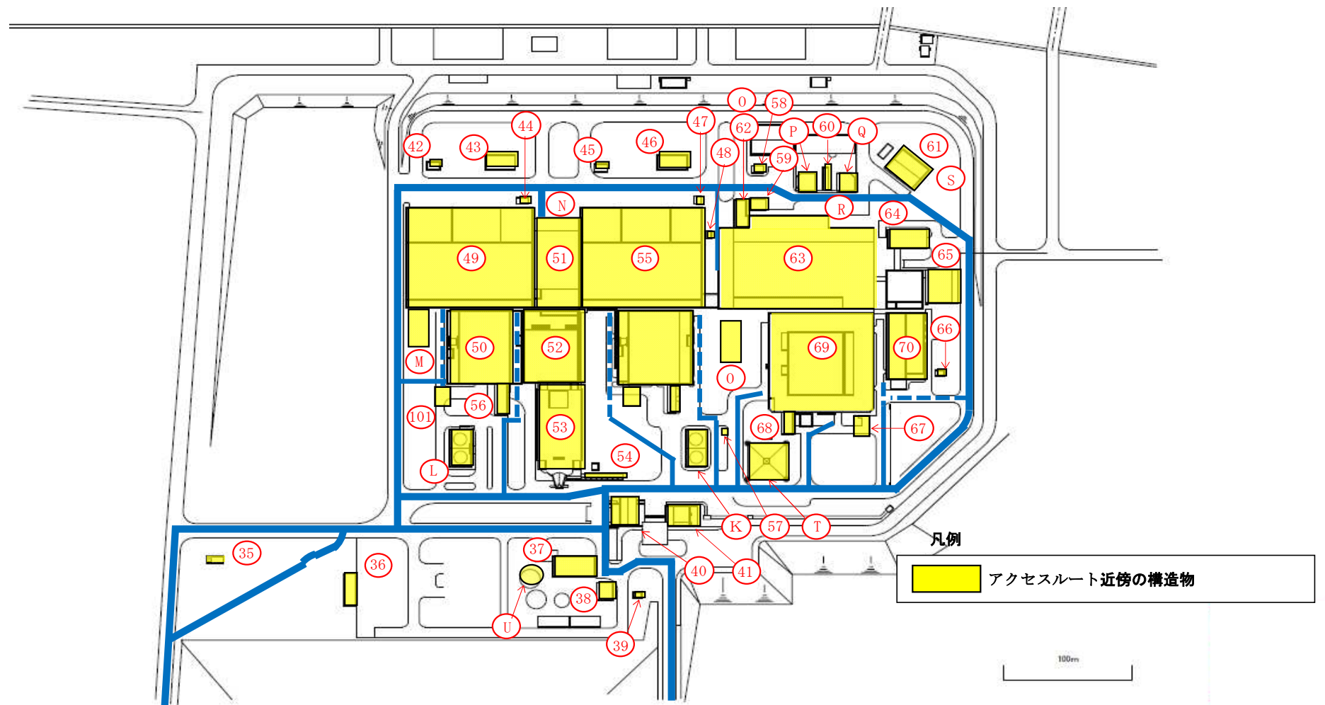
図 7-6 屋外アクセスルートの周辺構造物（大湊側詳細図）
