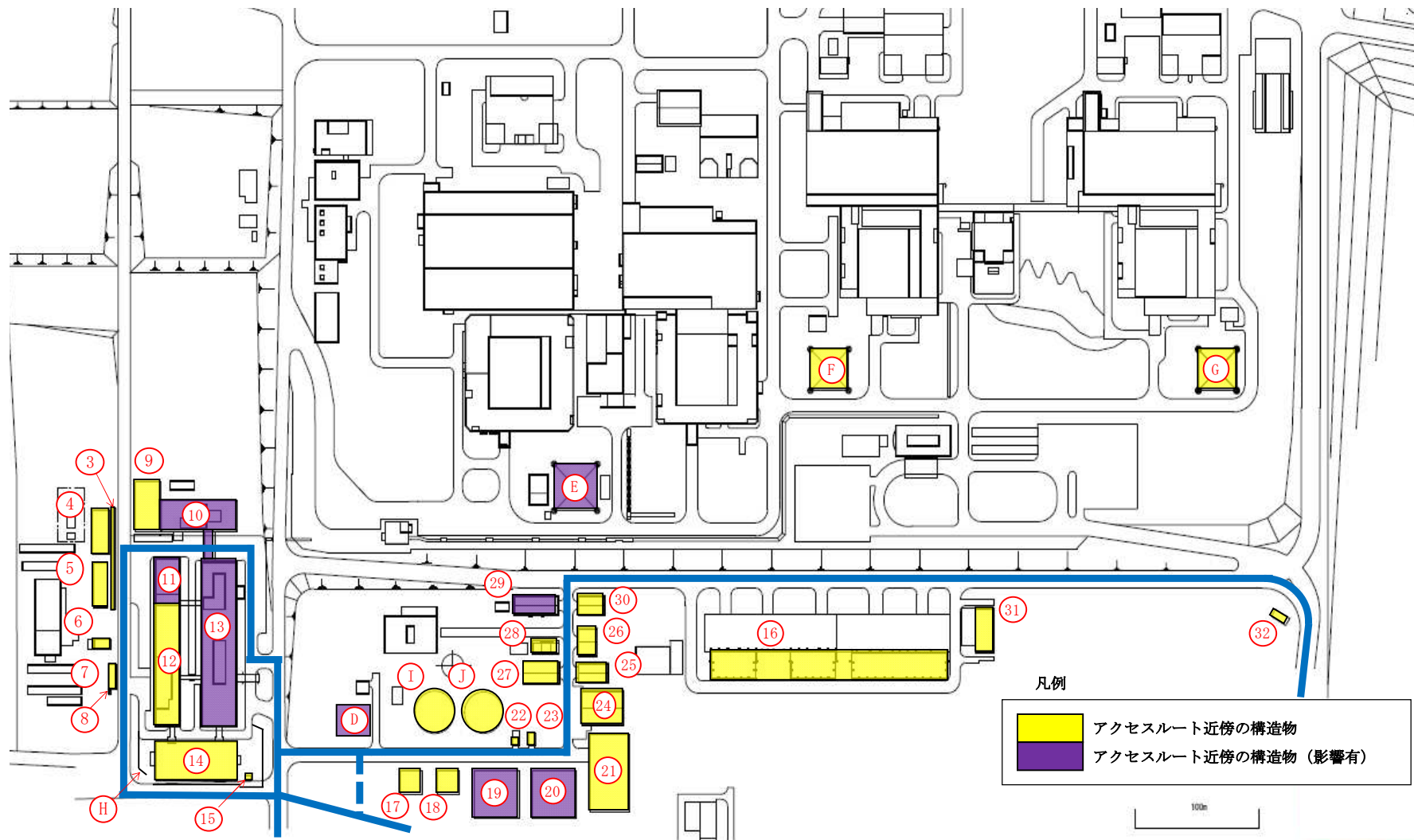
図 7-15 建屋倒壊時の屋外アクセスルートへの影響評価結果 (荒浜側詳細図)
