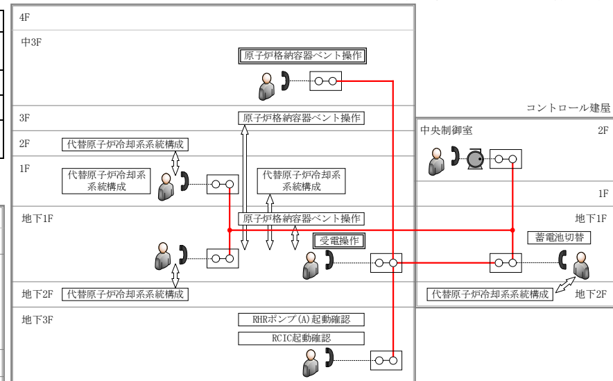
原子炉建屋
