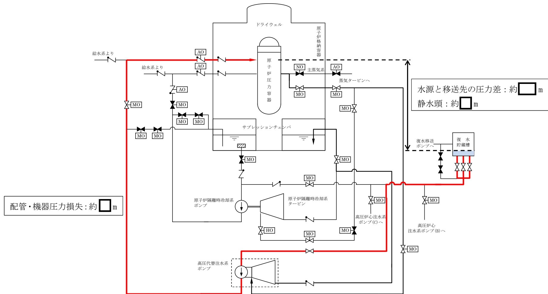
図1 高压代替注水系の系統概略図
