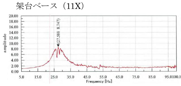
図 2-2(1) X 方向 周波数応答関数
