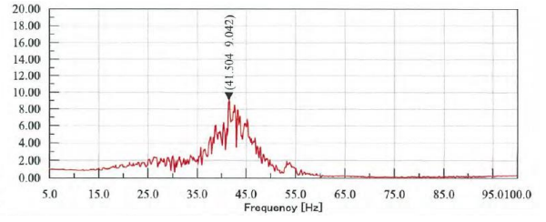
架台ベース (8Y)
