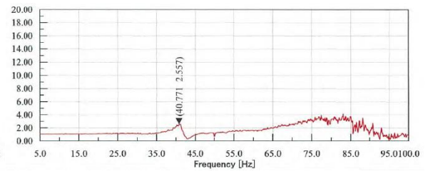
架台ベース (2Z)
