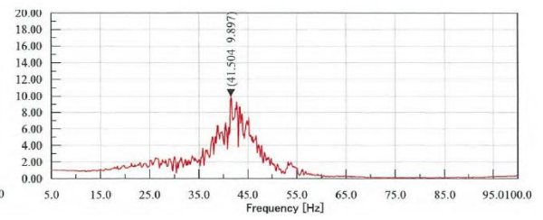
架台ベース (10Y)
