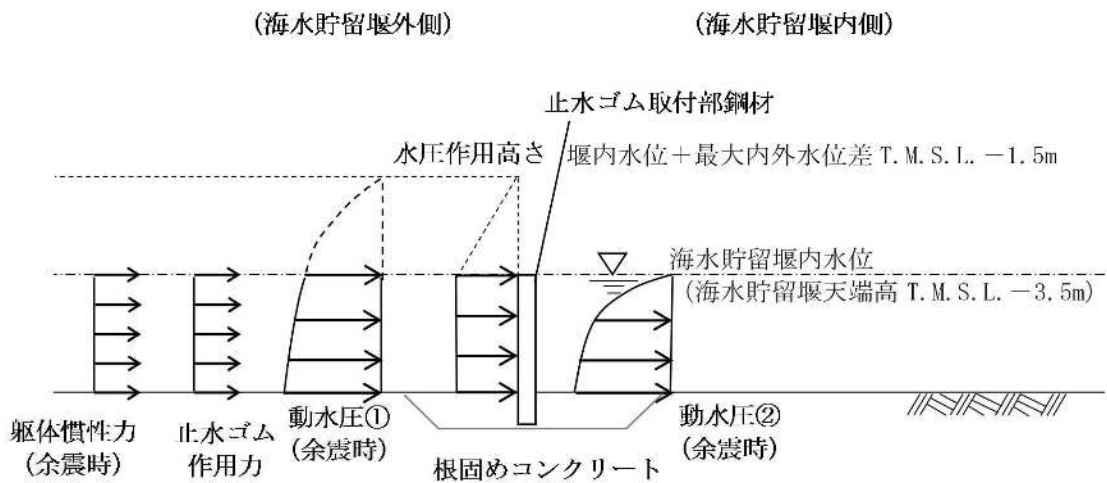
図 2.3-3-3 荷重作用図（止水ゴム取付部鋼材 重畳時 2）
