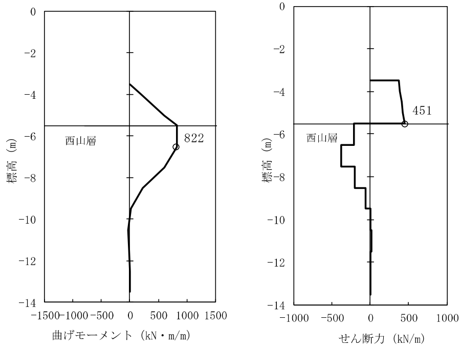
(a) 地盤ばね 1 (津波時)
