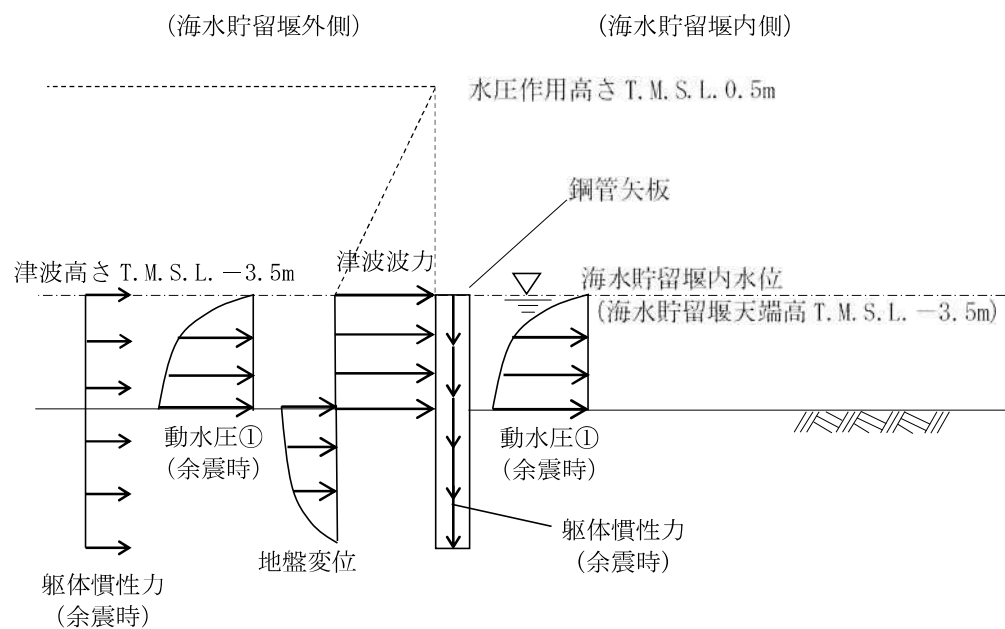
図 1.5-2 津波荷重+余震荷重が海水貯留堰に作用するイメージ図
