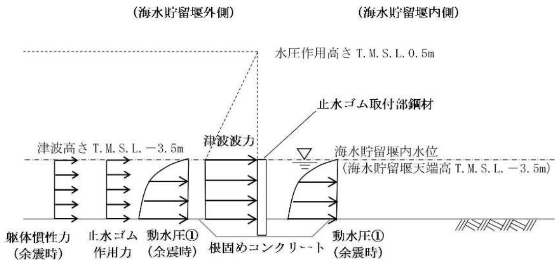
図 2.3-3-2 荷重作用図（止水ゴム取付部鋼材 重畳時 1）
