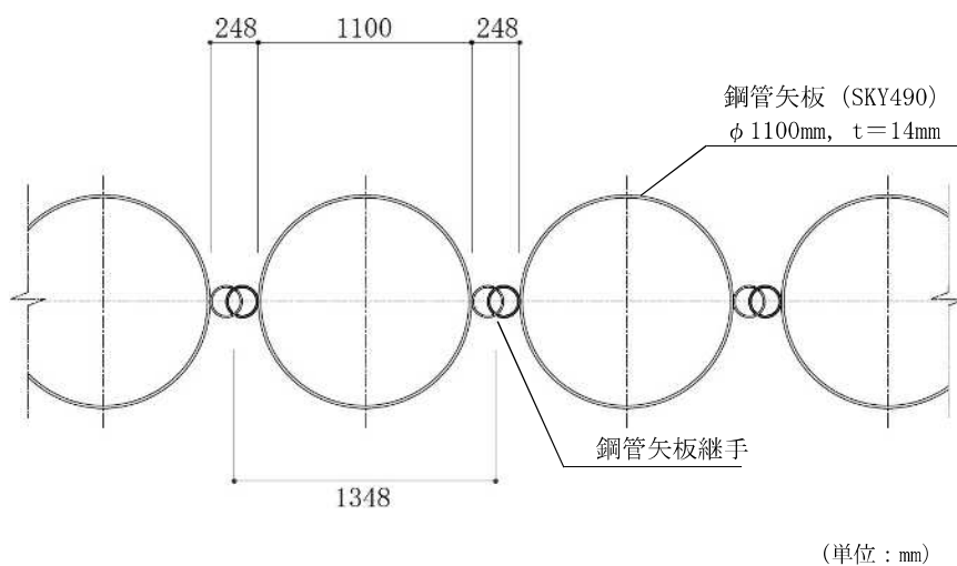
(a) 鋼管矢板 一般部
