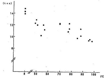
第 5-1 図 引張強度と温度の関係
