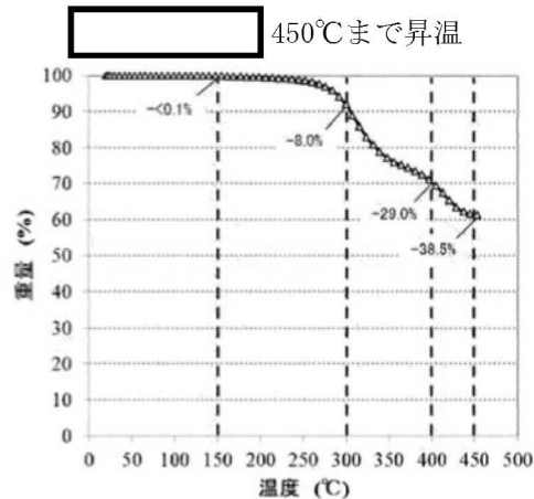
図 8-1 温度と重量減少の関係
