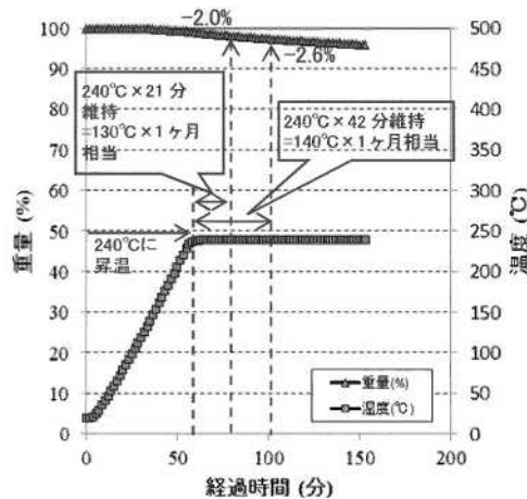
図 8-2 240°C 保持試験
