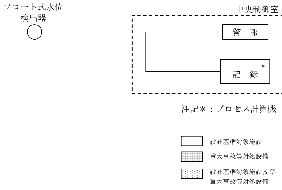
図3-3 使用済燃料貯蔵プール水位の概略構成図
