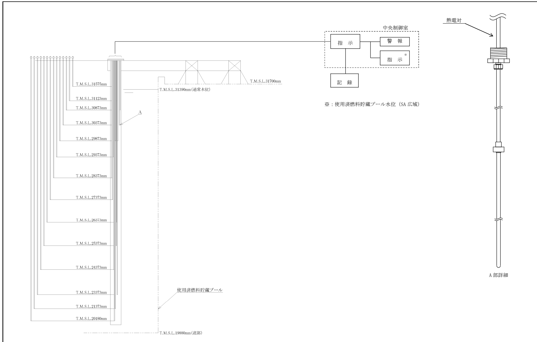
図 3-10 使用済燃料貯蔵プール水位・温度 (SA 広域) の構造図
