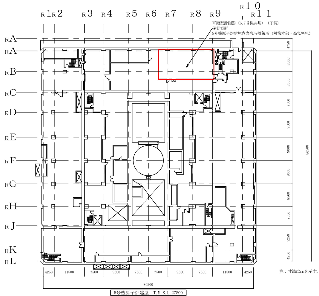
図 3-19 可搬型計測器 (6,7号機共用) (予備) の保管場所を明示した図面
