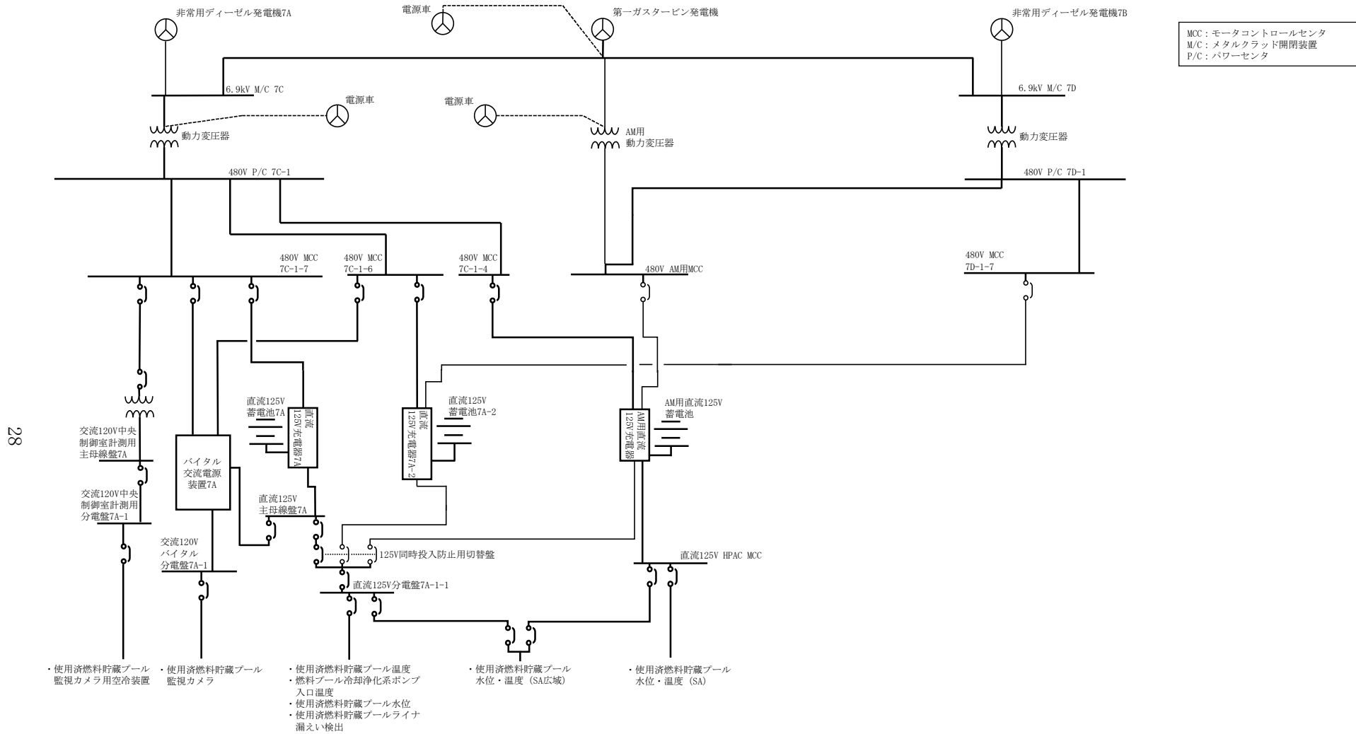
図 3-20 使用済燃料貯蔵プールの温度及び水位等を監視する装置の概略電源系統図
