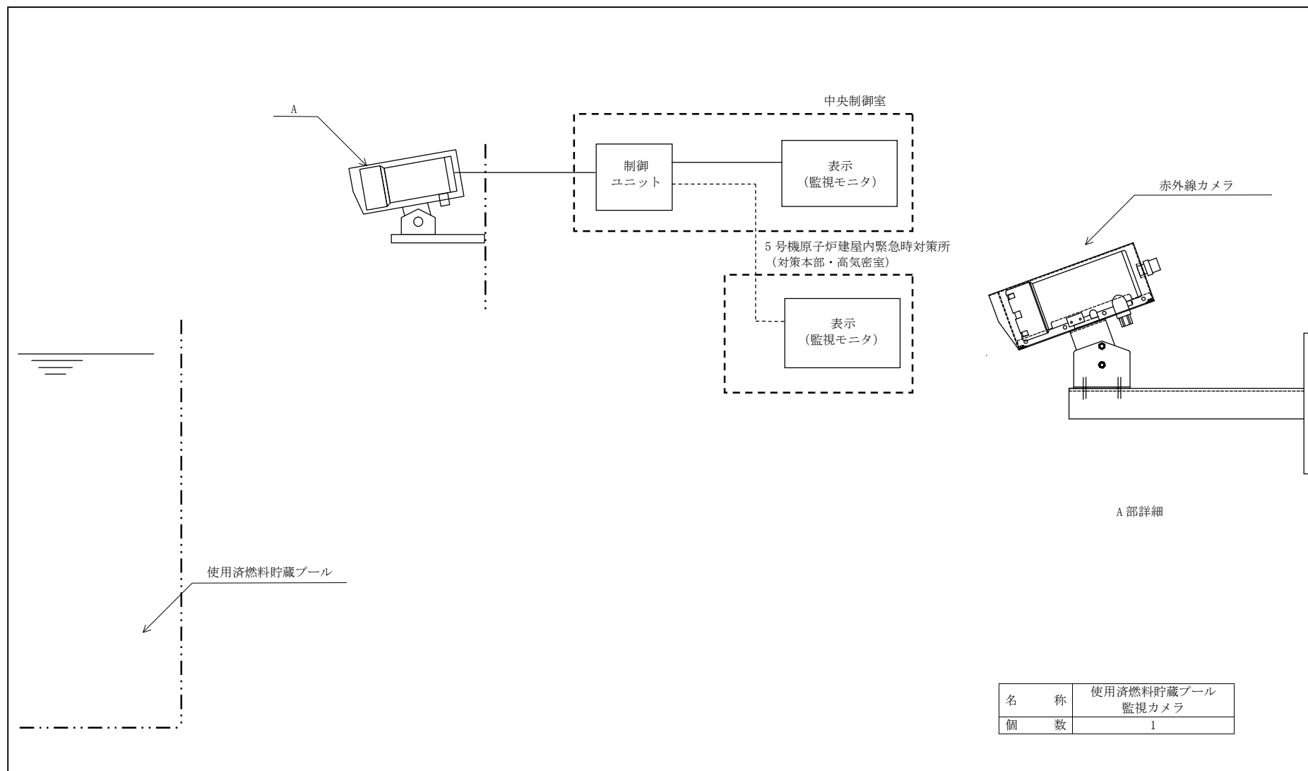
図 3-12 使用済燃料貯蔵プール監視カメラの構造図
