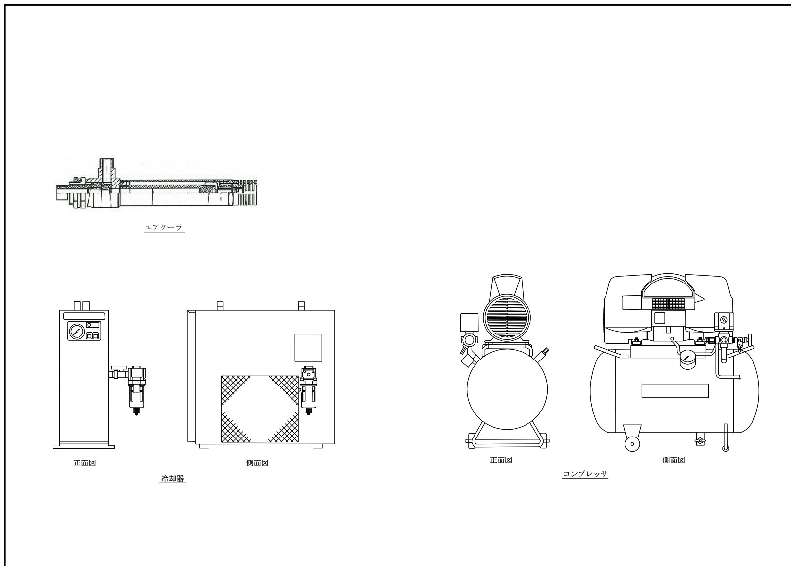
図 3-15 使用済燃料貯蔵プール監視カメラ用空冷装置の構造図
