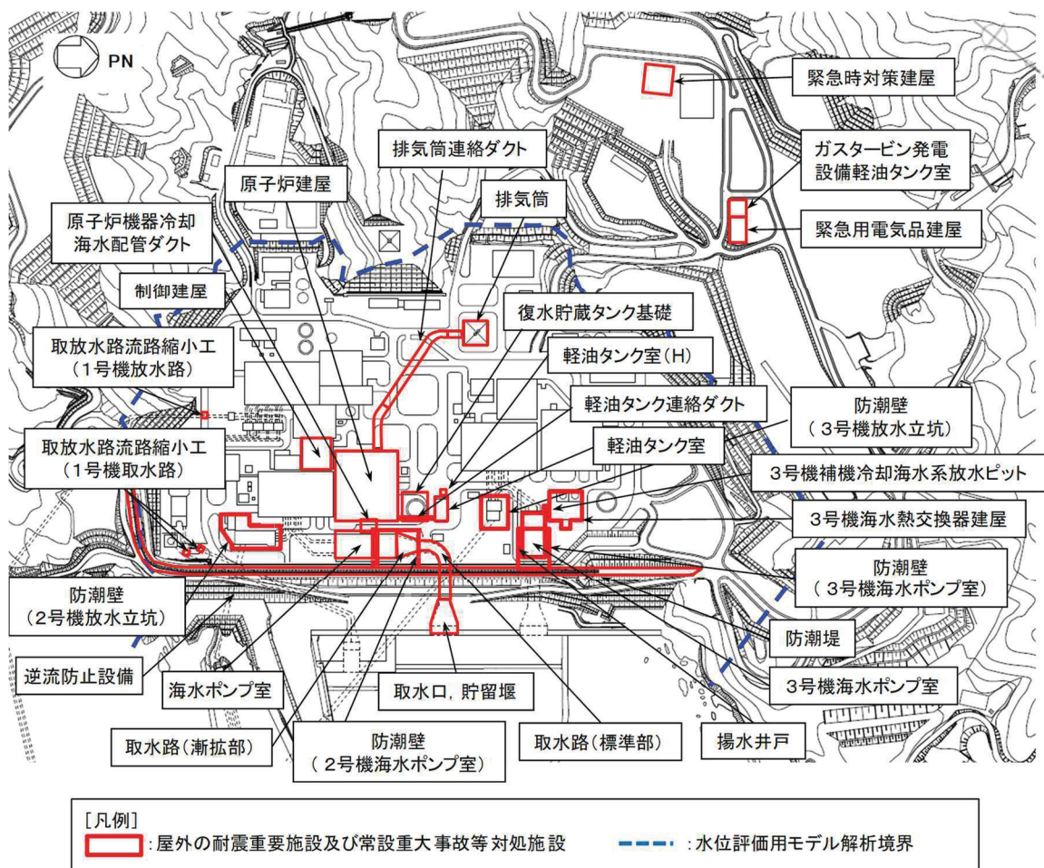
図3.3-6 屋外の評価対象施設の配置図
