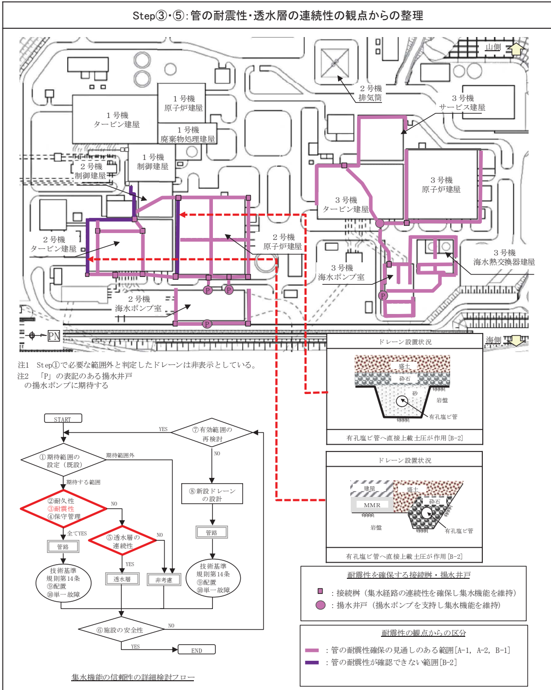
図 2-4-6 管の耐震性・透水層の連続性の観点からの整理結果 (Step③・⑤)
