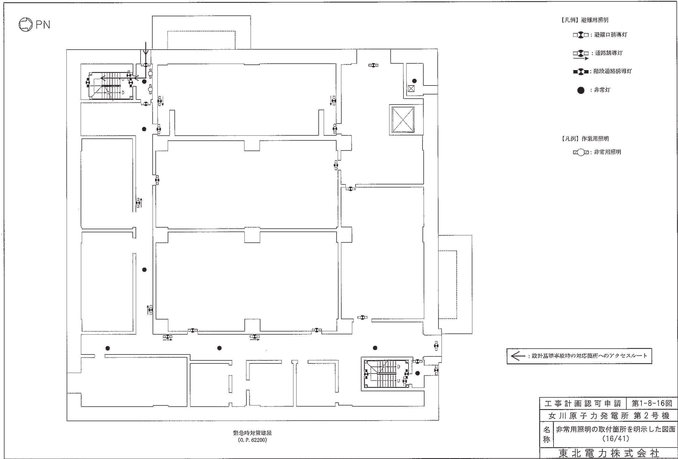
図4 作業用照明の設置場所及び中央制御室から各現場機器室までのアクセスルートの詳細 (11/11)
