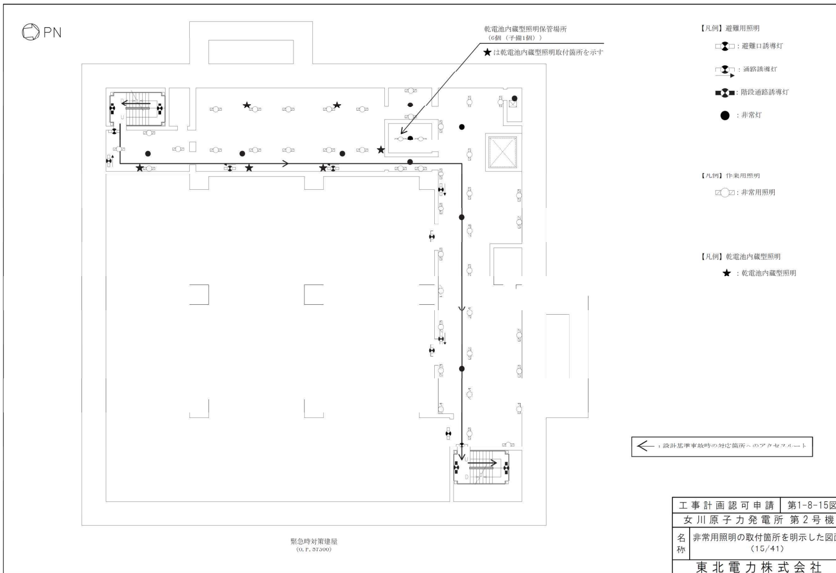
図4 作業用照明の設置場所及び中央制御室から各現場機器室までのアクセスルートの詳細 (10/11)
