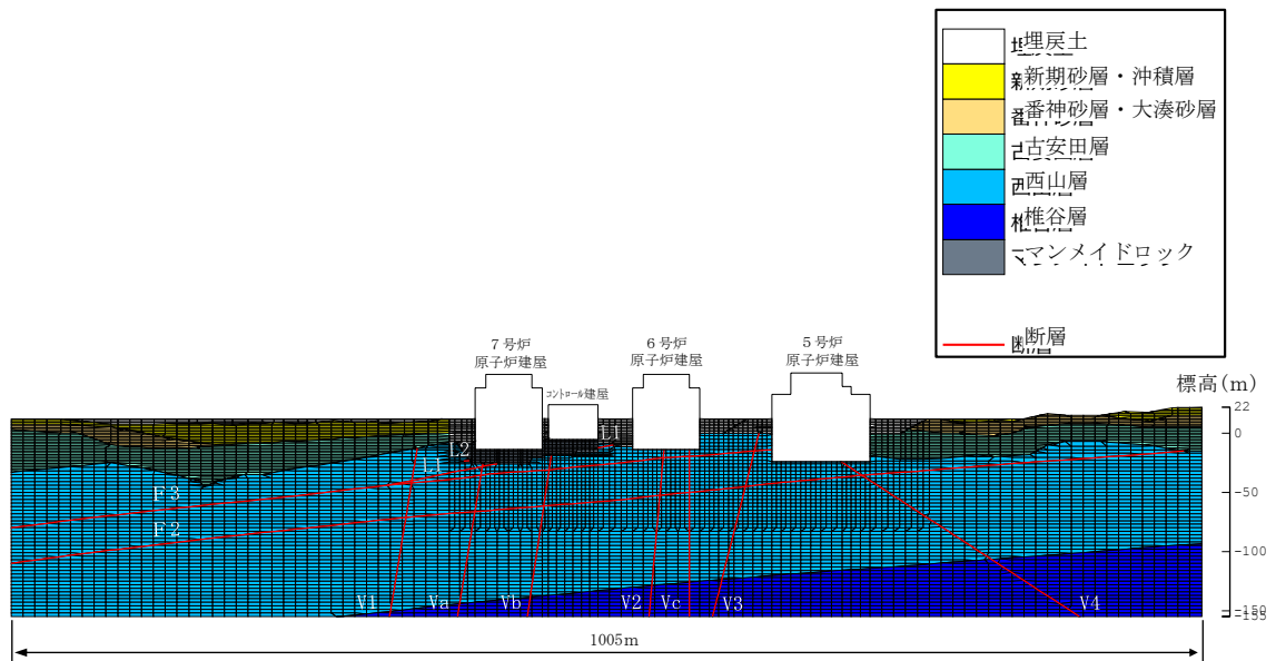
図-2 解析用要素分割図 (5号、6号及び7号機原子炉建屋汀線平行断面)
