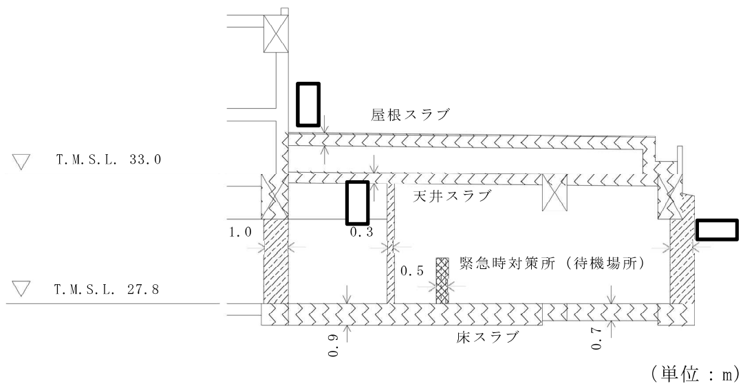
C-C 断面
