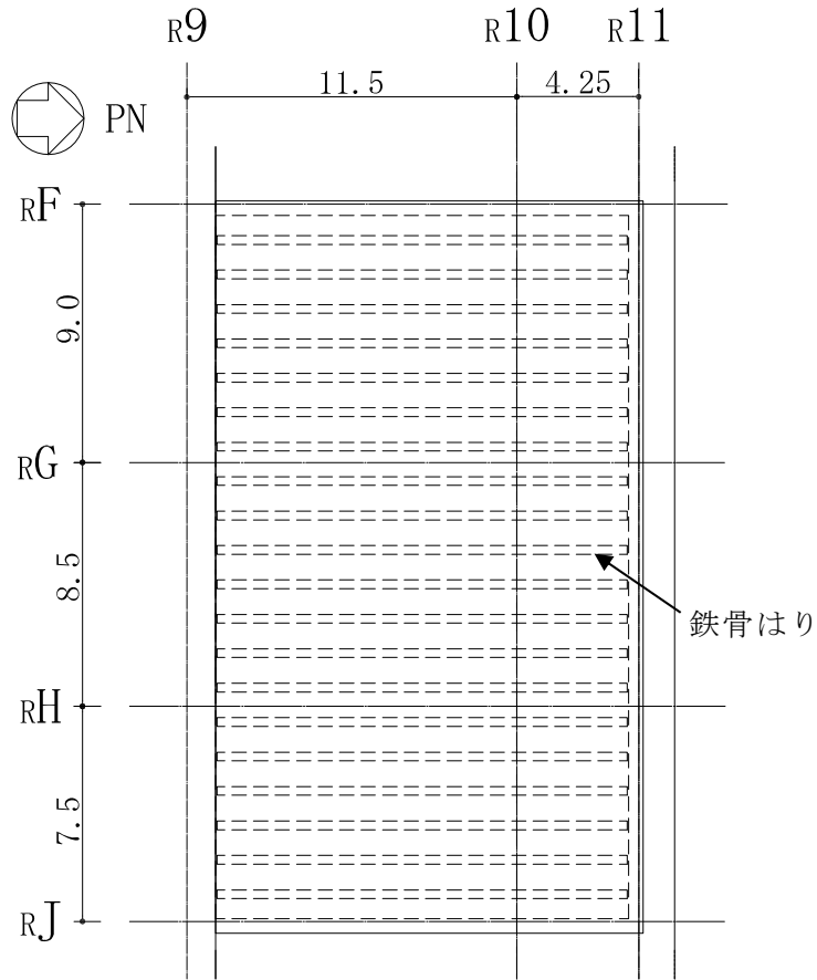
(c) 緊急時対策所 (対策本部) 屋根スラブ
