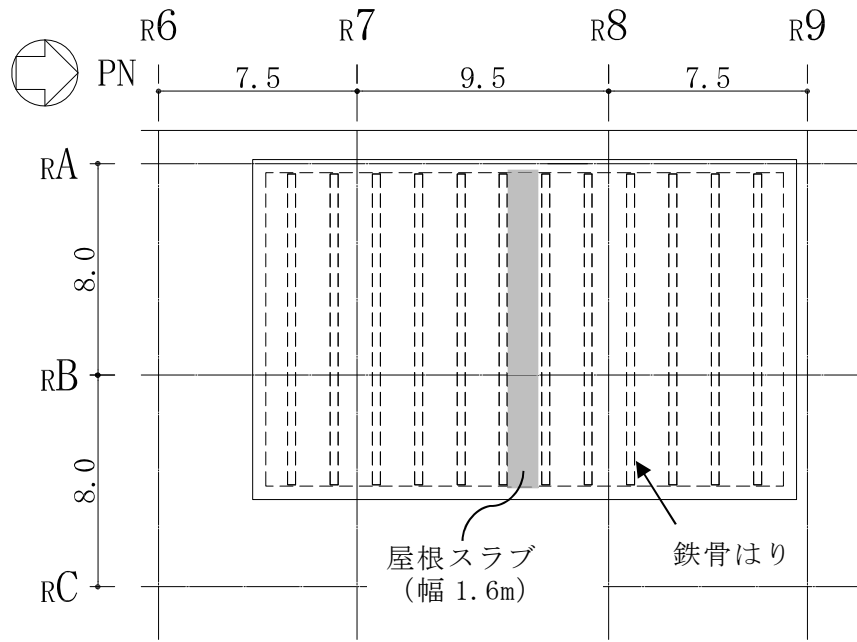
(c) 緊急時対策所 (対策本部) 屋根スラブ
