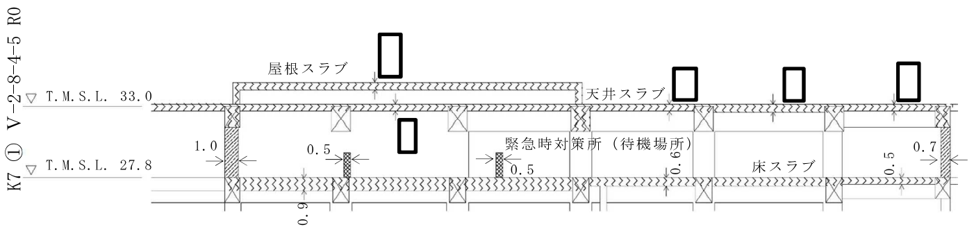
D-D 断面
