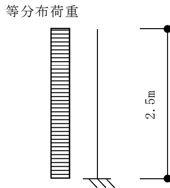
図 4-8 解析モデル
