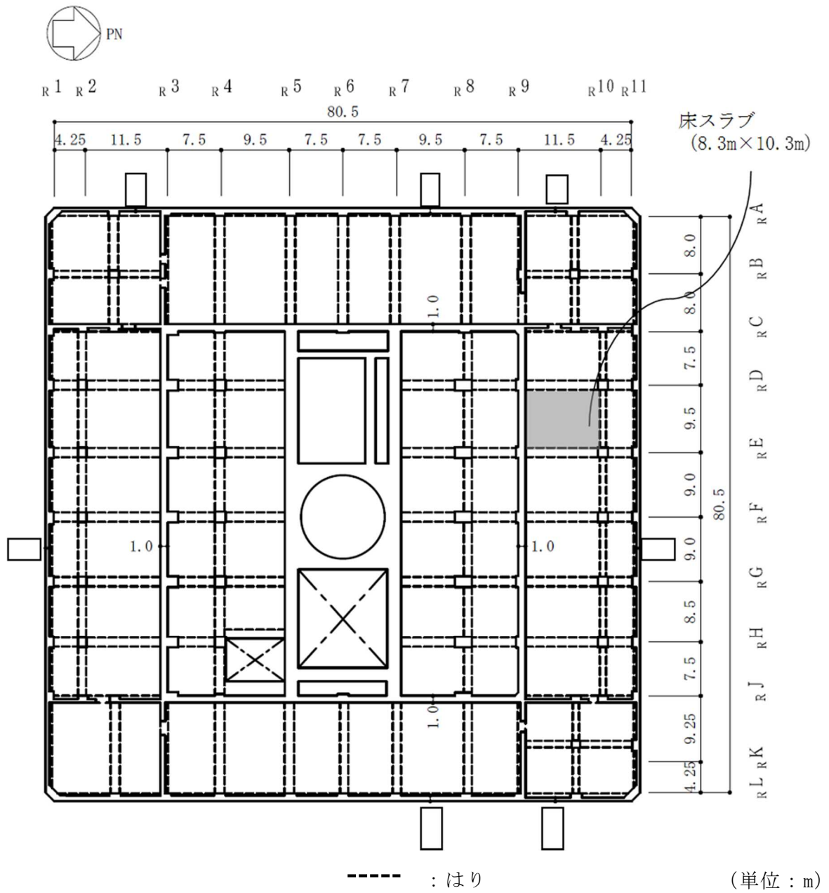
(a) 緊急時対策所 床スラブ
