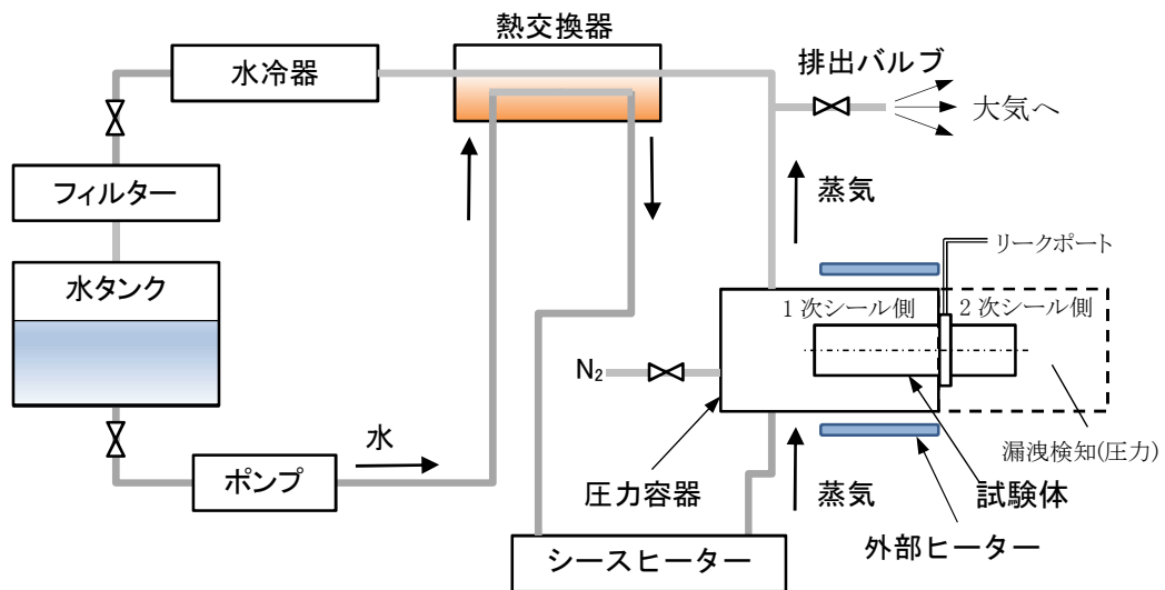
図 2 試験装置の系統概略図
