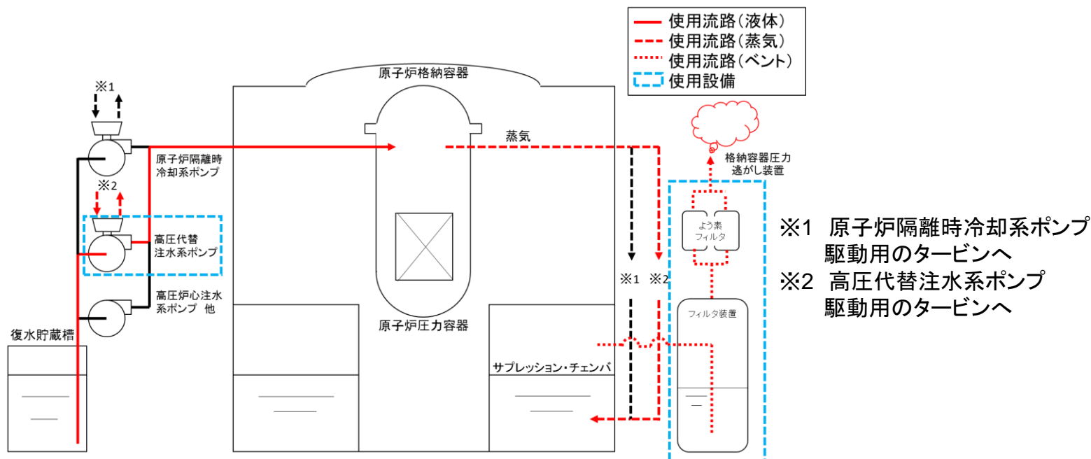
図2-2. 高圧代替注水系使用時の系統図
