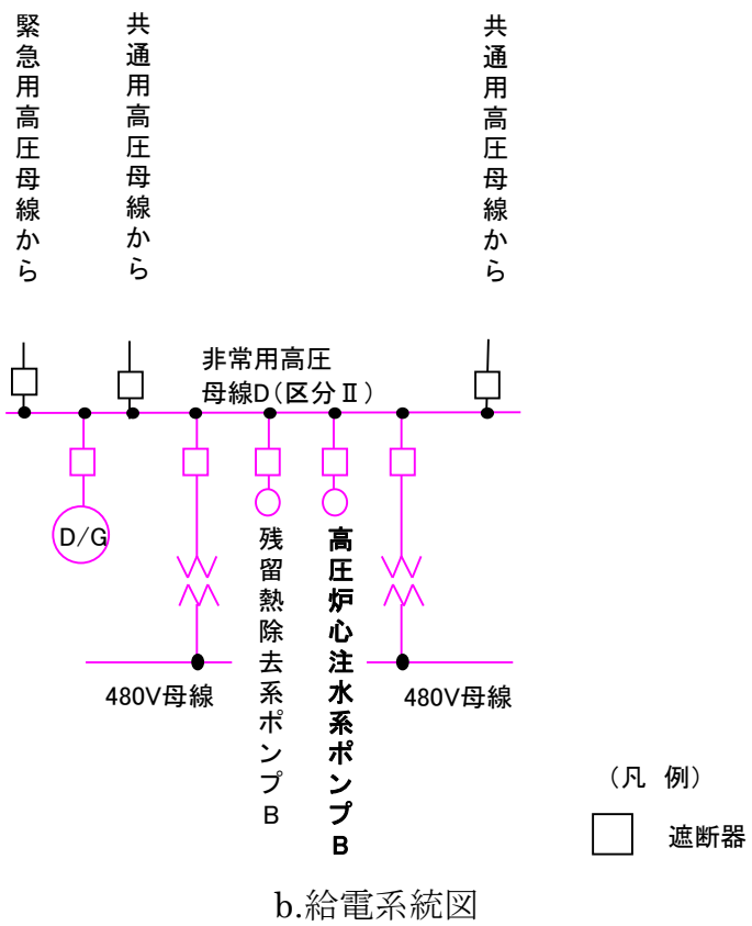
第6図 対策の概略系統図 (非常用ディーゼル発電機の機能維持) (イの対応)
