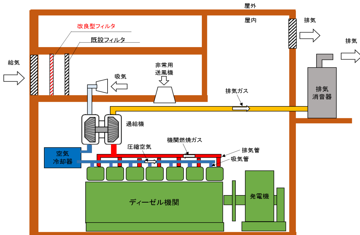
図2-1. フィルタ外形図 及び非常用ディーゼル発電機の給気ライン概略図
