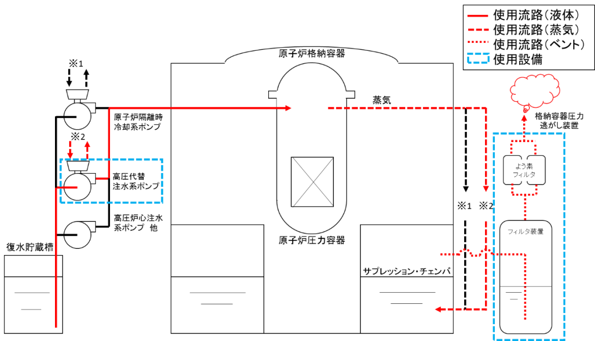
a.系統図
