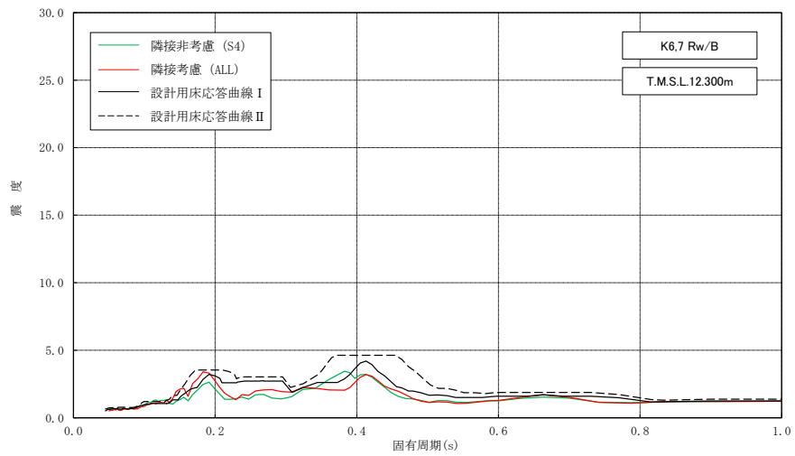
図 3-42 床応答スペクトルの比較 (Rw/B, 水平方向, 減衰 2.0%) (2/3)
