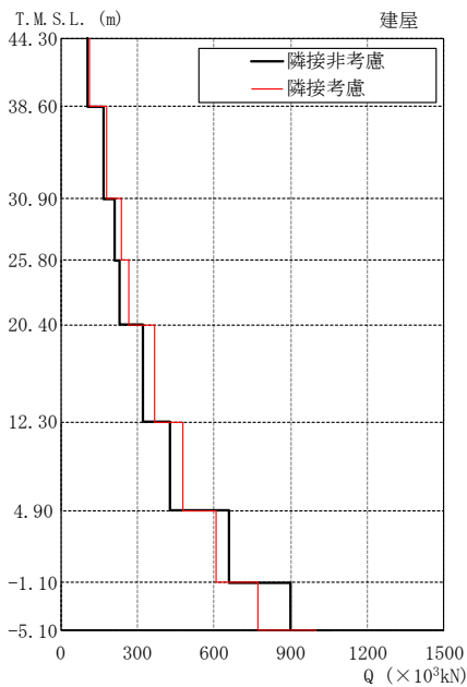
図 3-15 最大応答せん断力の比較 (K7T/B, EW 方向)
