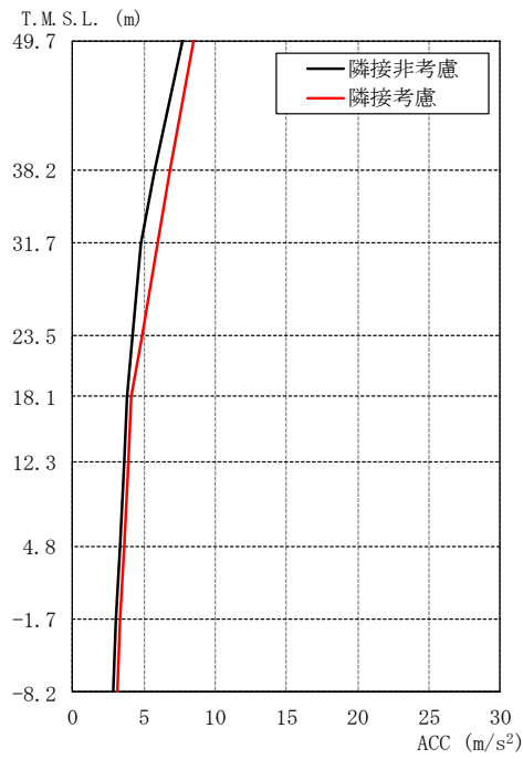
図 3-2 最大応答加速度の比較 (K7R/B, NS 方向)
