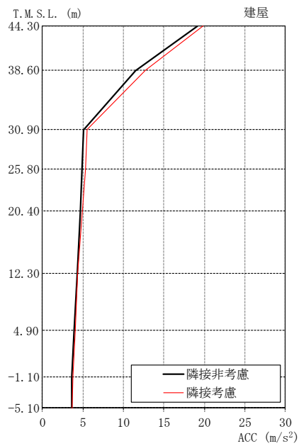
図 3-13 最大応答加速度の比較 (K7T/B, EW 方向)
