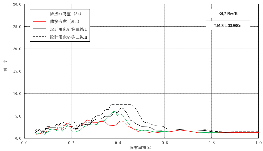
図 3-42 床応答スペクトルの比較 (Rw/B, 水平方向, 減衰 2.0%) (1/3)
