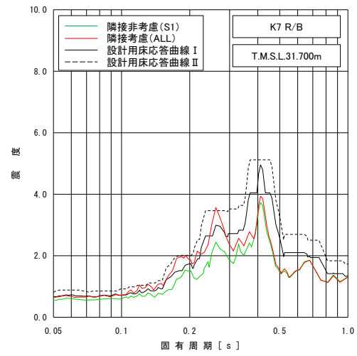
図 3-39 床応答スペクトルの比較 (K7R/B, 水平方向, 減衰 2.0%) (1/3)
