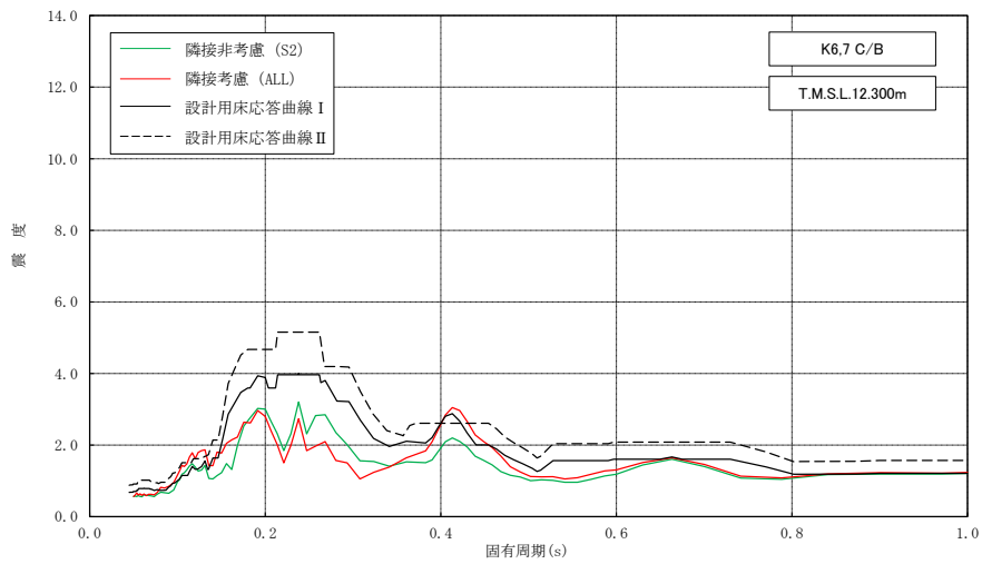
図 3-40 床応答スペクトルの比較 (C/B, 水平方向, 減衰 2.0%) (1/2)
