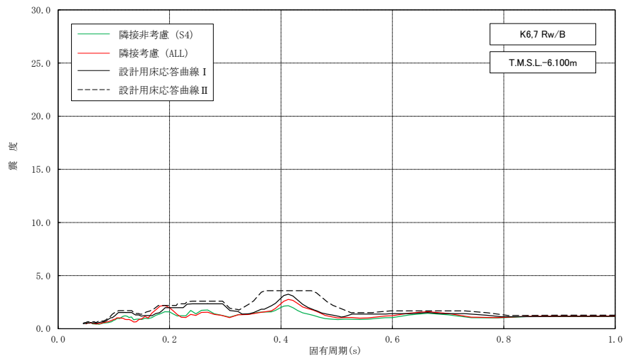
図 3-42 床応答スペクトルの比較 (Rw/B, 水平方向, 減衰 2.0%) (3/3)
