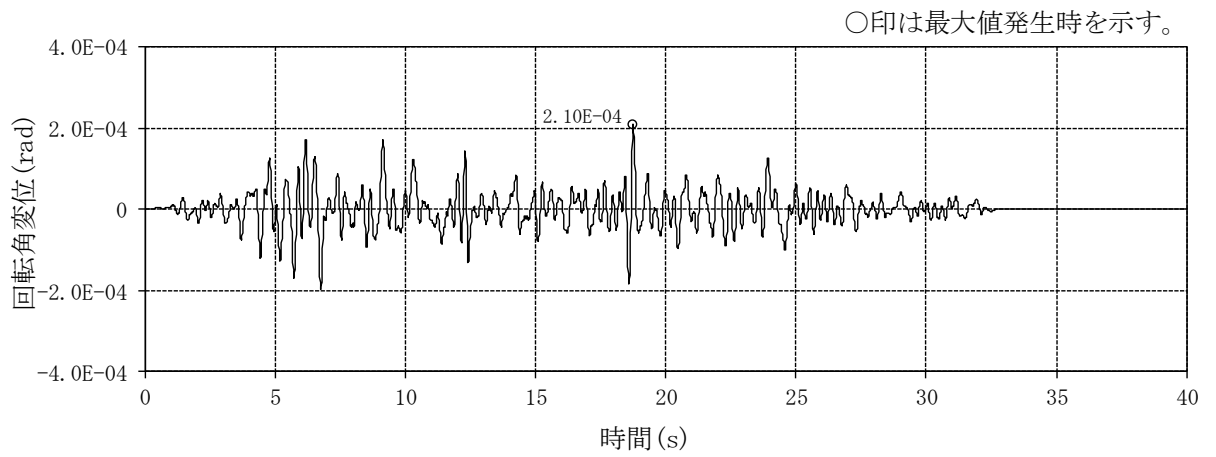
(b) 回転角変位
