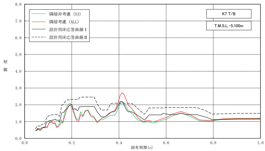
図 3-41 床応答スペクトルの比較 (K7T/B, 水平方向, 減衰 2.0%) (3/3)
