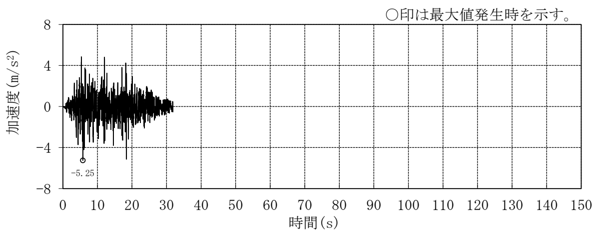
図 3-14 検討用地震動 S_d-1H
