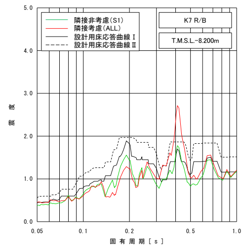
図 3-39 床応答スペクトルの比較 (K7R/B, 水平方向, 減衰 2.0%) (3/3)
