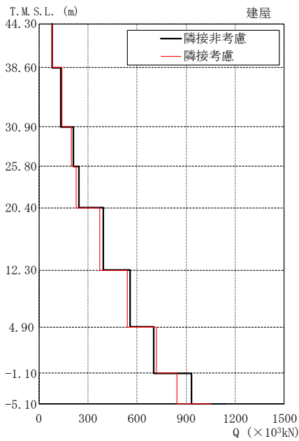
図 3-14 最大応答せん断力の比較 (K7T/B, NS 方向)
