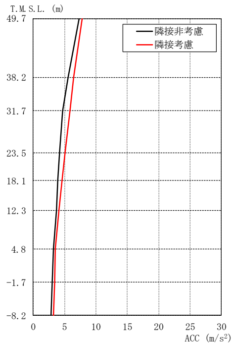
図 3-3 最大応答加速度の比較 (K7R/B, EW 方向)
