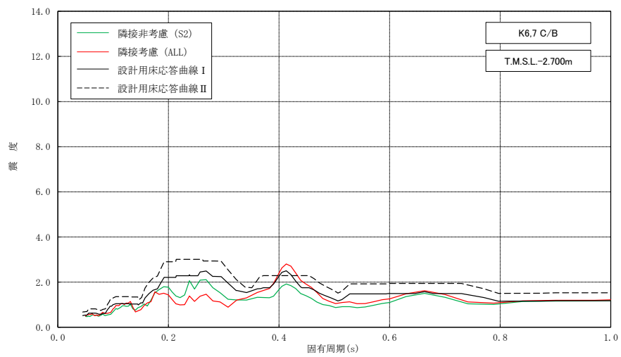
図 3-40 床応答スペクトルの比較 (C/B, 水平方向, 減衰 2.0%) (2/2)
