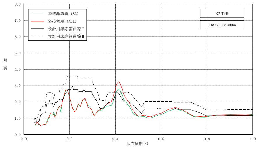
図 3-41 床応答スペクトルの比較 (K7T/B, 水平方向, 減衰 2.0%) (2/3)
