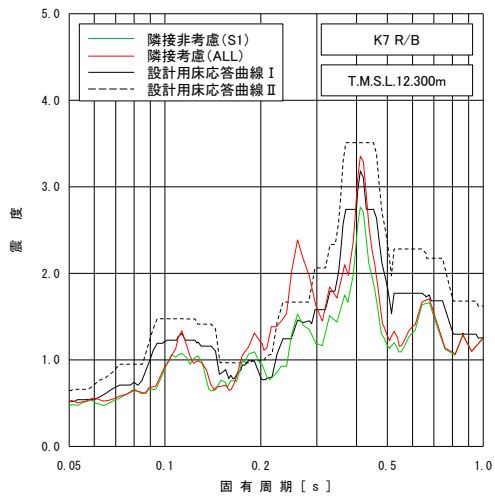
図 3-39 床応答スペクトルの比較 (K7R/B, 水平方向, 減衰 2.0%) (2/3)
