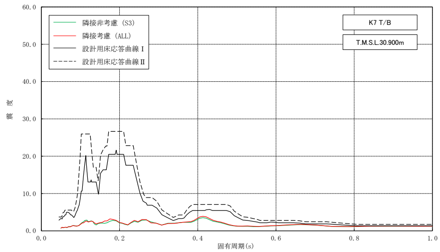
図 3-41 床応答スペクトルの比較 (K7T/B, 水平方向, 減衰 2.0%) (1/3)
