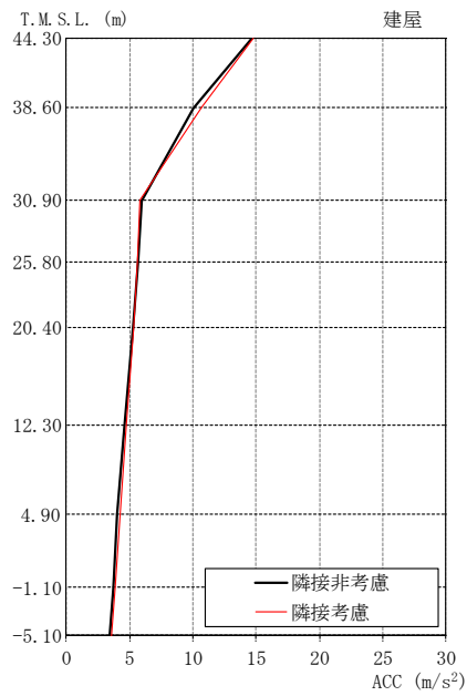
図 3-12 最大応答加速度の比較 (K7T/B, NS 方向)
