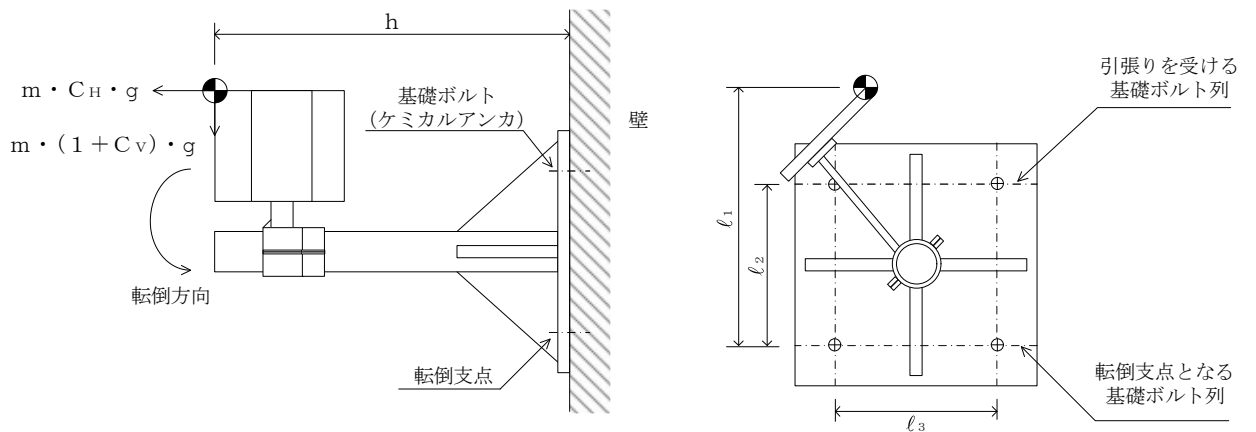
図5-2 計算モデル（側面方向転倒）
