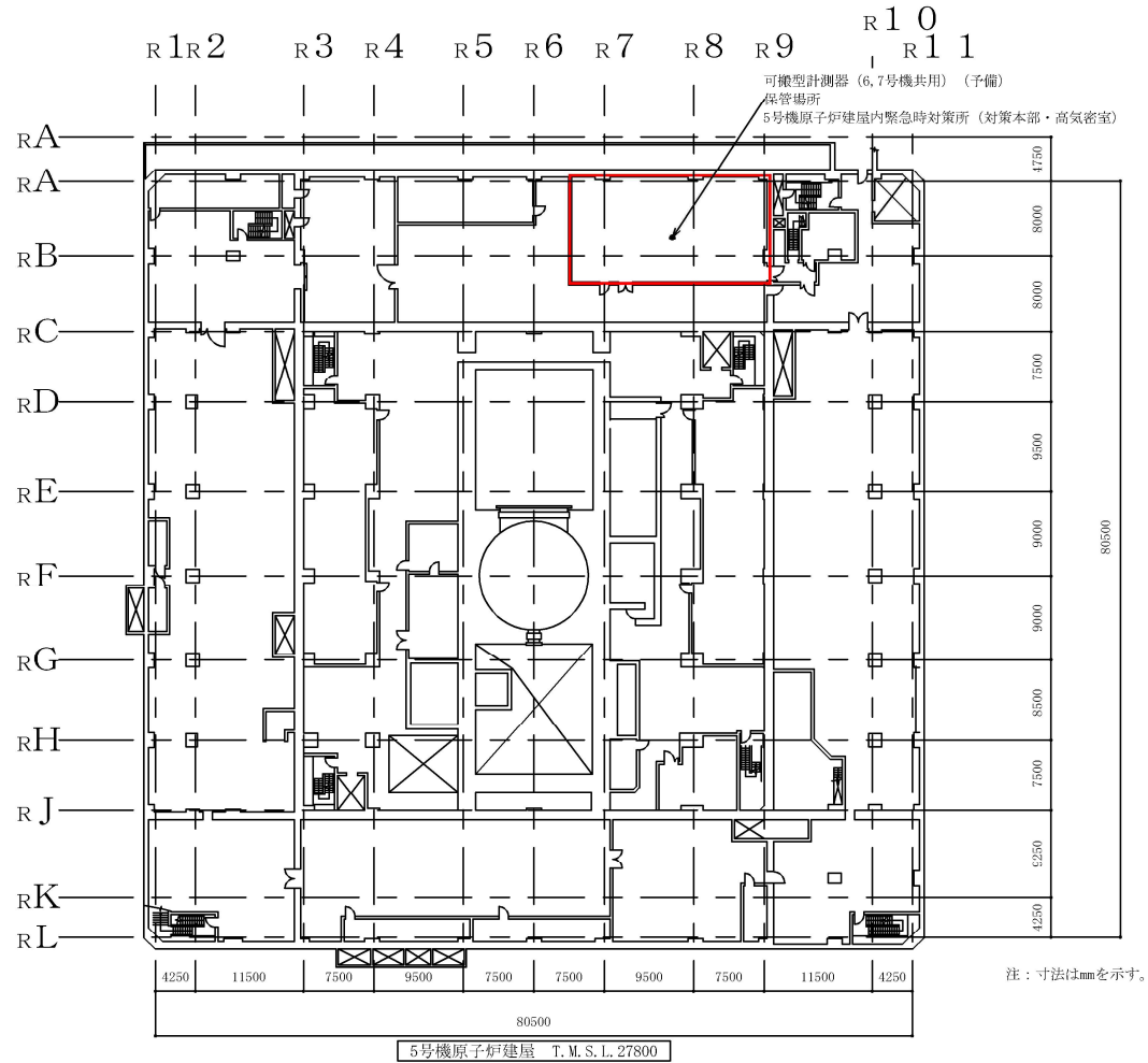
図 3-19 可搬型計測器 (6,7号機共用) (予備) の保管場所を明示した図面
