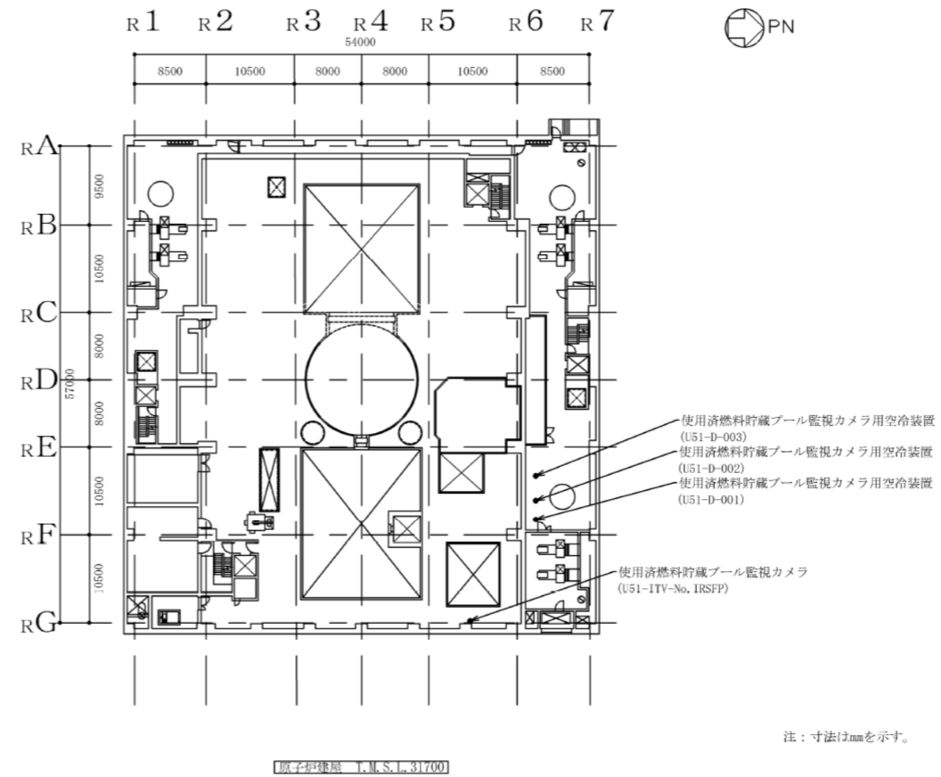
図 3-13 使用済燃料貯蔵プール監視カメラ及び使用済燃料貯蔵プール監視カメラ用空冷装置の取付箇所を明示した図面
