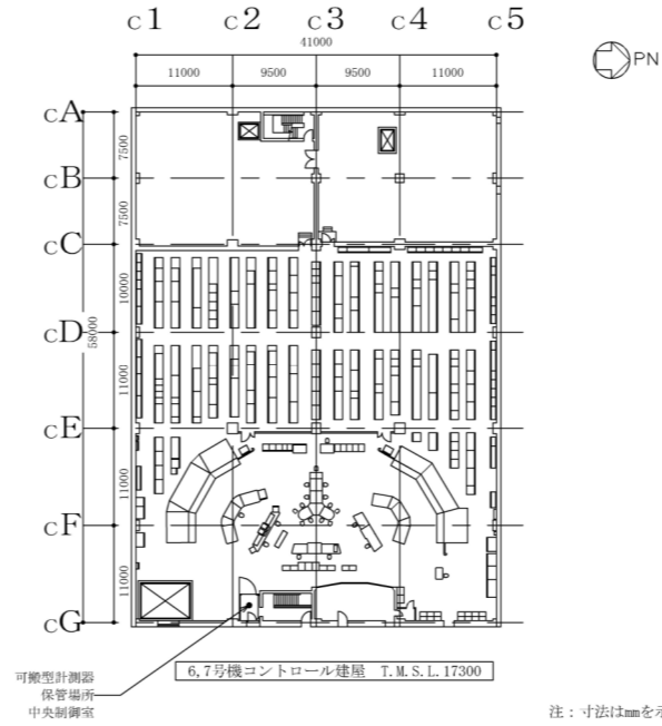
図3-18 可搬型計測器の保管場所を明示した図面
