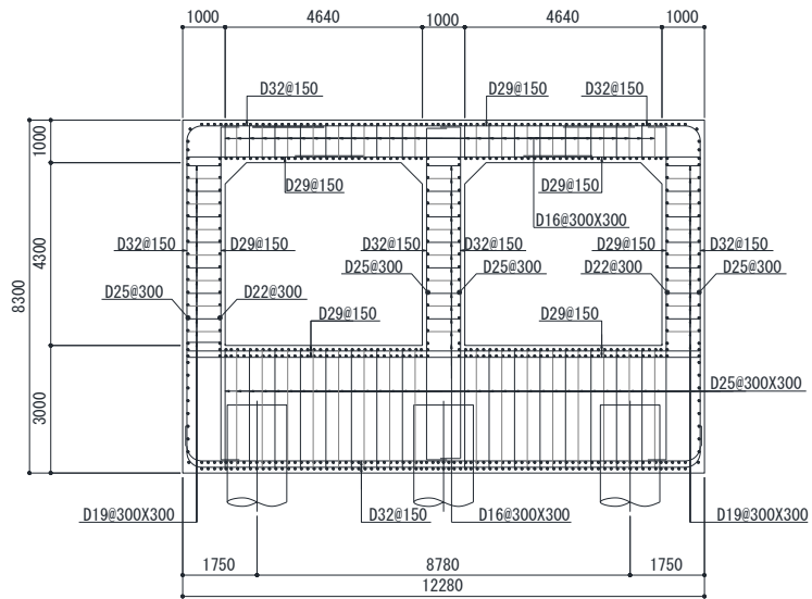
図 2-6 (2) 常設代替交流電源設備基礎の概略配筋図 (B-B断面)
