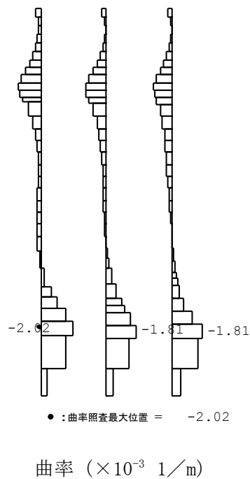
図 6-6 鋼管杭において最も厳しい照査値の曲率分布 (B-B断面) (解析ケース①, 地震動 Ss-3-, t=37.49s)
