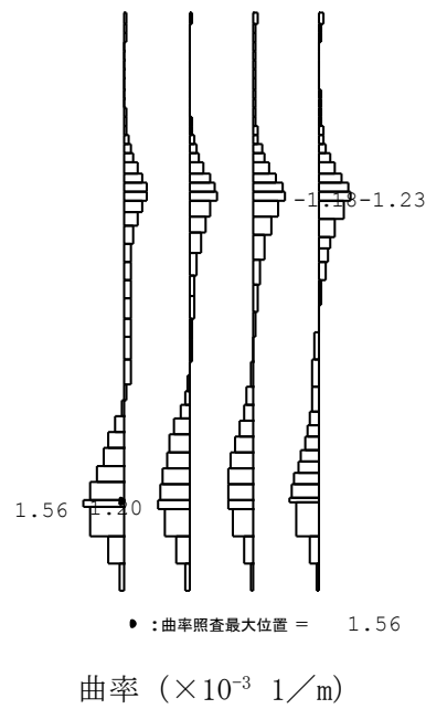
図 6-5 鋼管杭において最も厳しい照査値の曲率分布 (A-A断面) (解析ケース②, 地震動 Ss-3+, t=36.62s)
