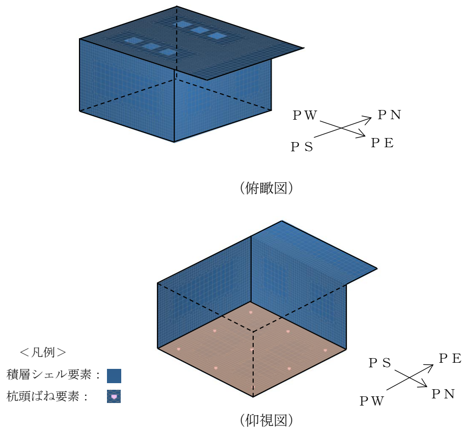
図 4-4 第一ガスタービン発電機用燃料タンク基礎モデル概念図
