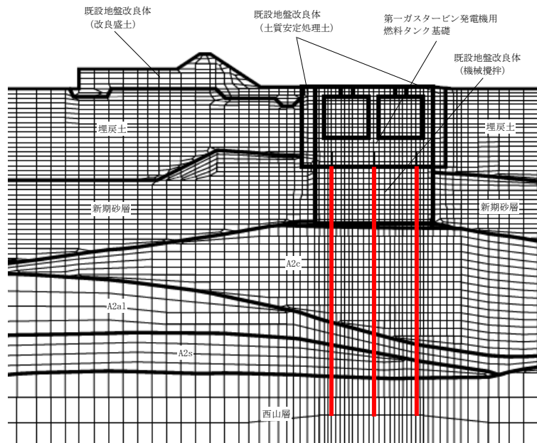
(B-B断面)
