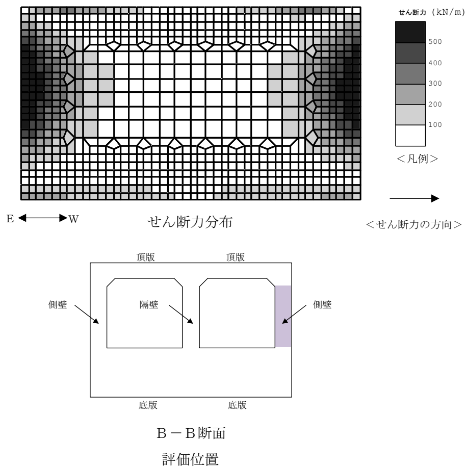
図 6-4 (2) 鉄筋コンクリート部材のせん断力照査が最も厳しくなるケースでの断面力分布図 (第一ガスタービン発電機用燃料タンク基礎(側壁③), 解析ケース③, 地震動 Ss-3ーー, t=17.34s)
