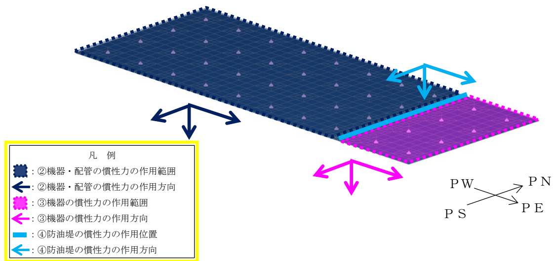
(a) 第一ガスタービン発電機基礎
