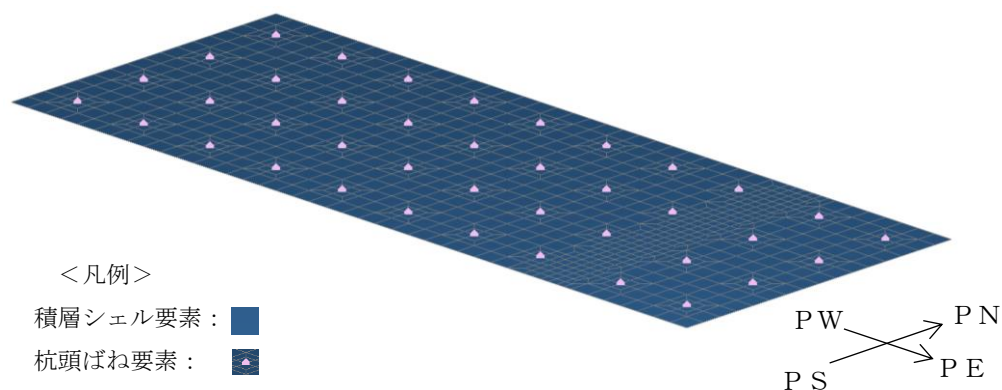
図 4-1 第一ガスタービン発電機基礎モデル概念図
