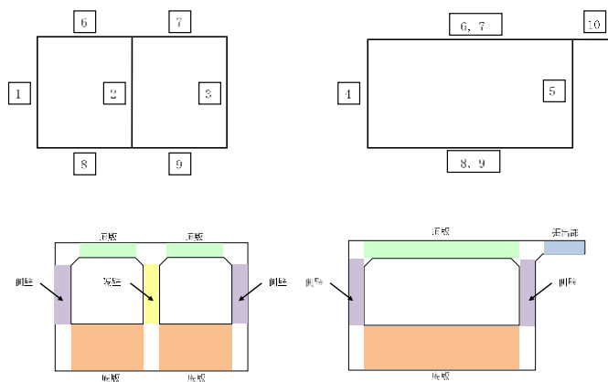
B-B断面
