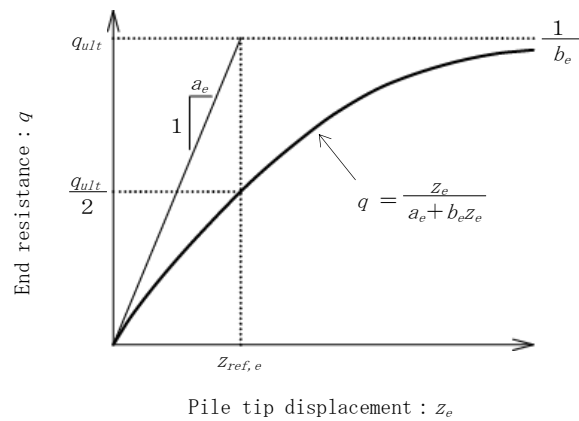
図 3-18 杭先端ばねの杭軸方向のばねの抵抗力と変位差関係 (Hirayama(1990))
