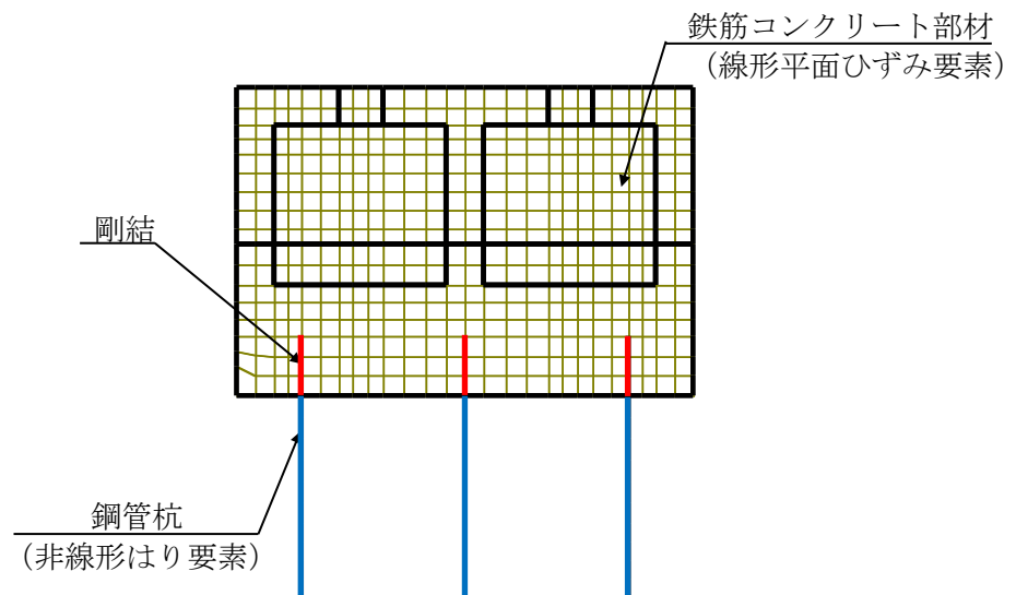
(a) 第一ガスタービン発電機基礎 (A-A断面, 構造物部分拡大部)
