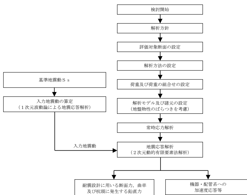
図 2-8 常設代替交流電源設備基礎の地震応答解析フロー
