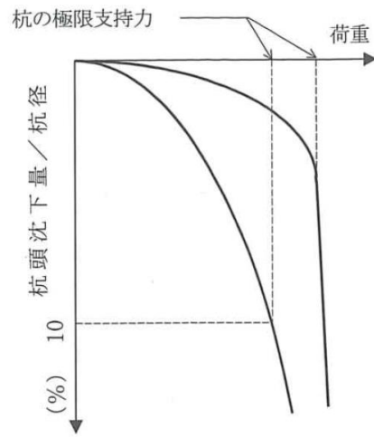
図 3-17 杭の鉛直載荷試験における一般的な荷重－変位関係 (道路橋示方書より引用)
