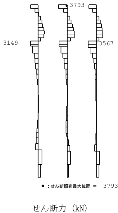
図 6-9 鋼管杭において最も厳しい照査値の地震時せん断力分布 (B-B断面) (解析ケース①, 地震動 Ss-3++, t=17.89s)
