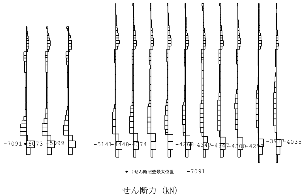
図 6-10 鋼管杭において最も厳しい照査値の地震時せん断力分布 (C-C断面) (解析ケース③, 地震動 Ss-3+, t=37.48s)
