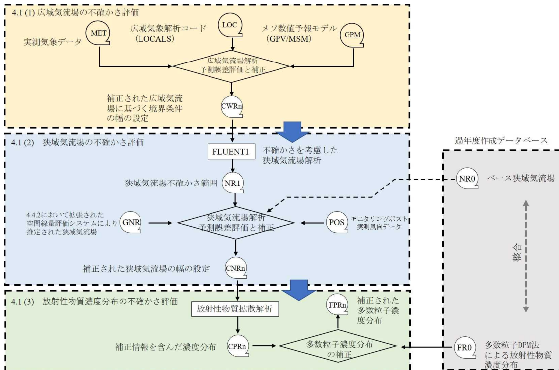
図 4.2 気流場及び放射性物質濃度分布の不確かさを考慮するためのデータベース構造の評価例
